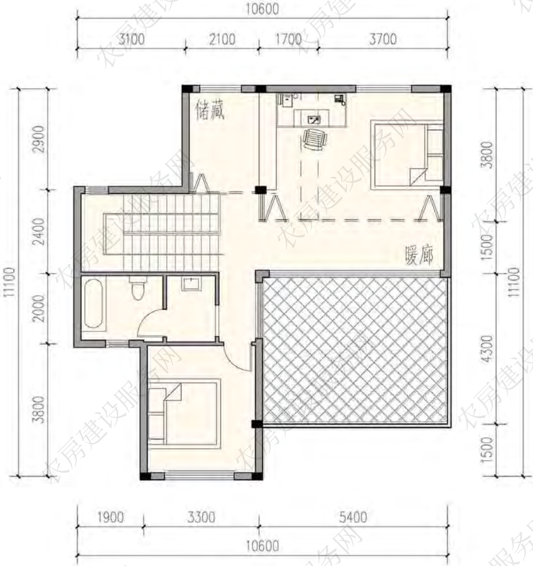
二层平面图
