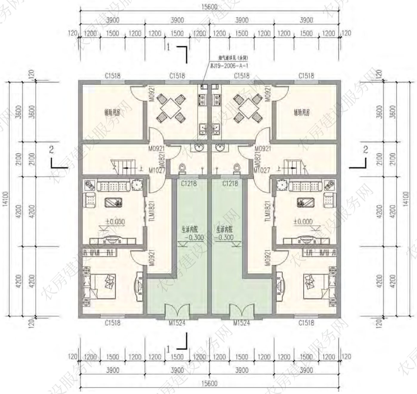
一层平面图
