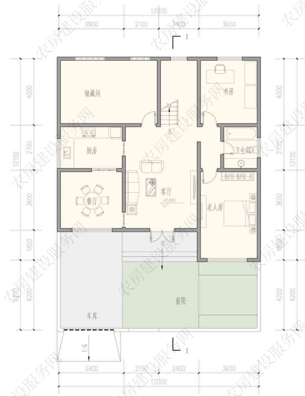
一层平面图
