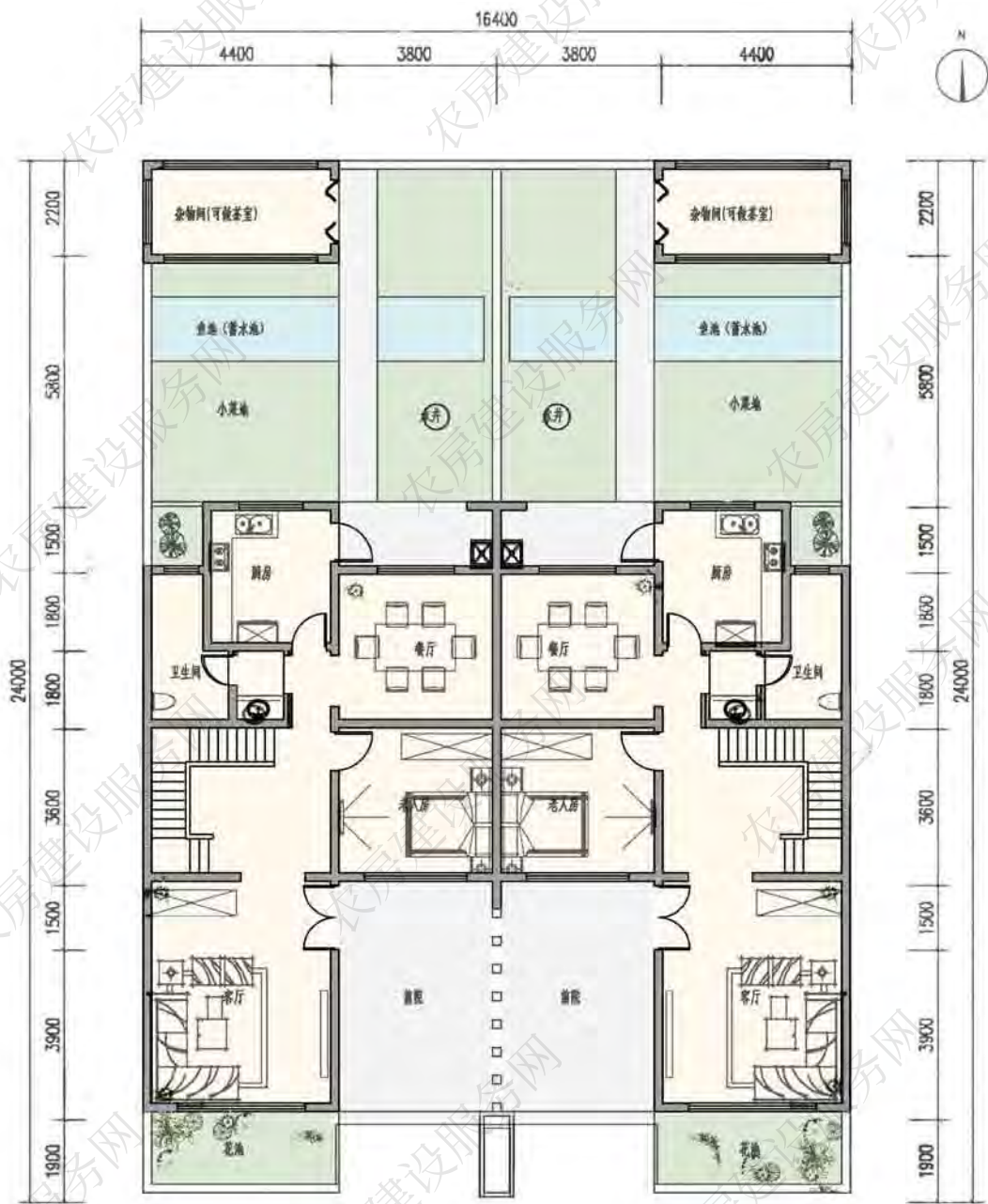
一层平面图
