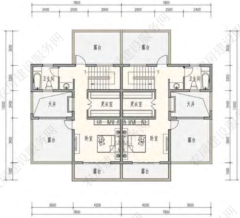
三层平面图
