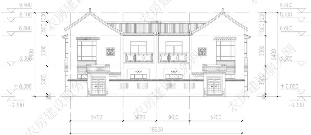
南立面图
