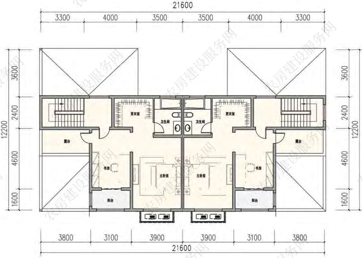
三层平面图
