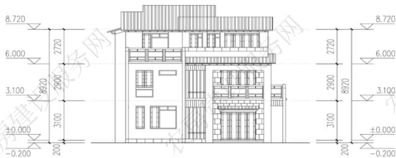
南立面图
