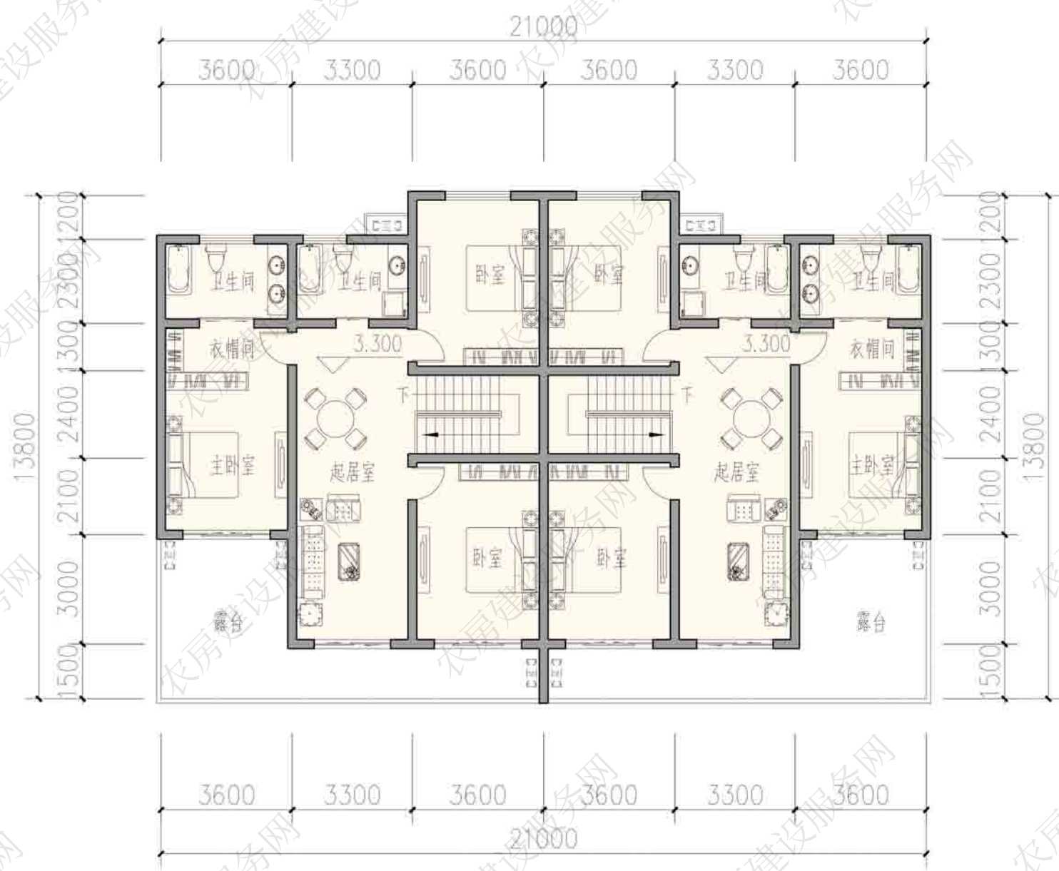
二层平面图
