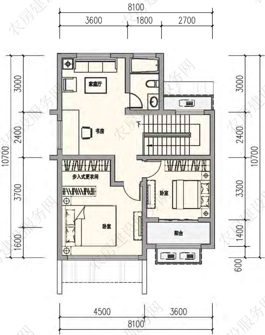
二层平面图
