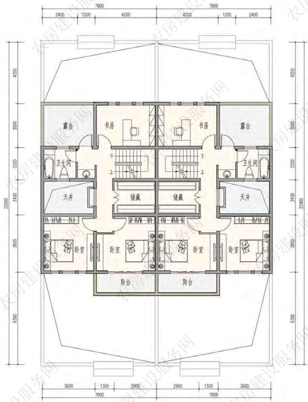
二层平面图
