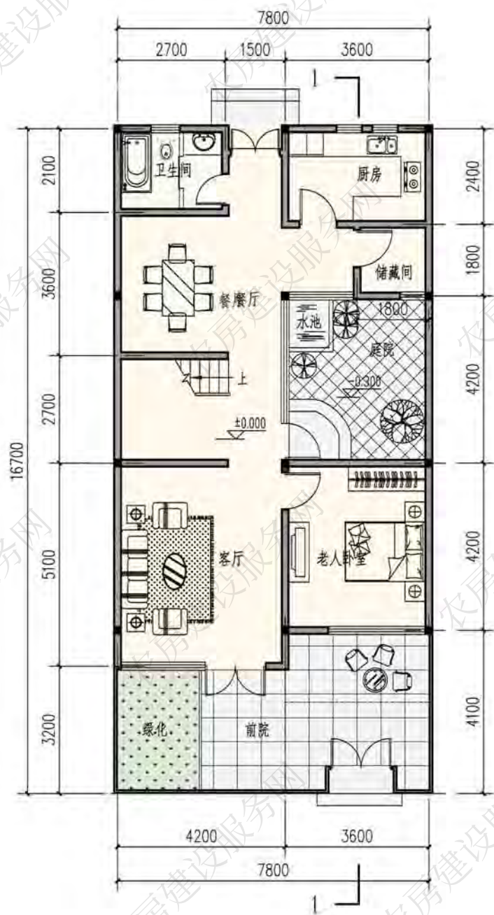
一层平面图
