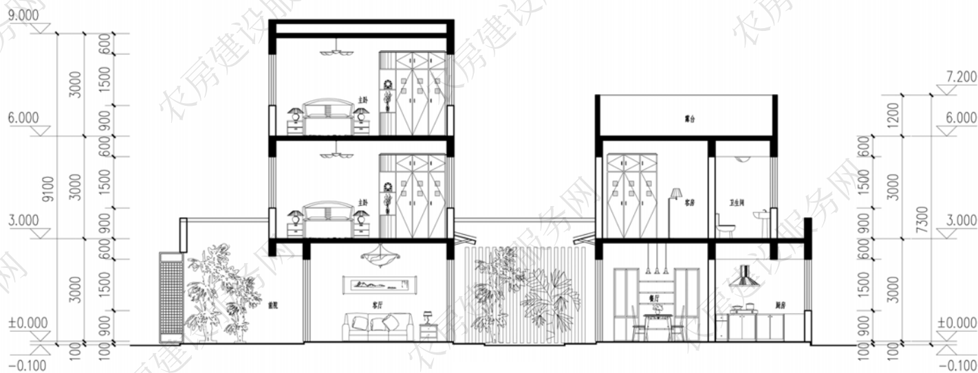
1-1 剖面图
