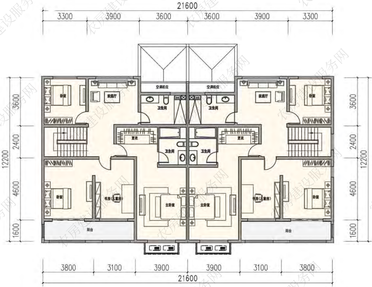
二层平面图
