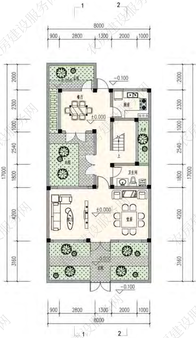
一层平面图
