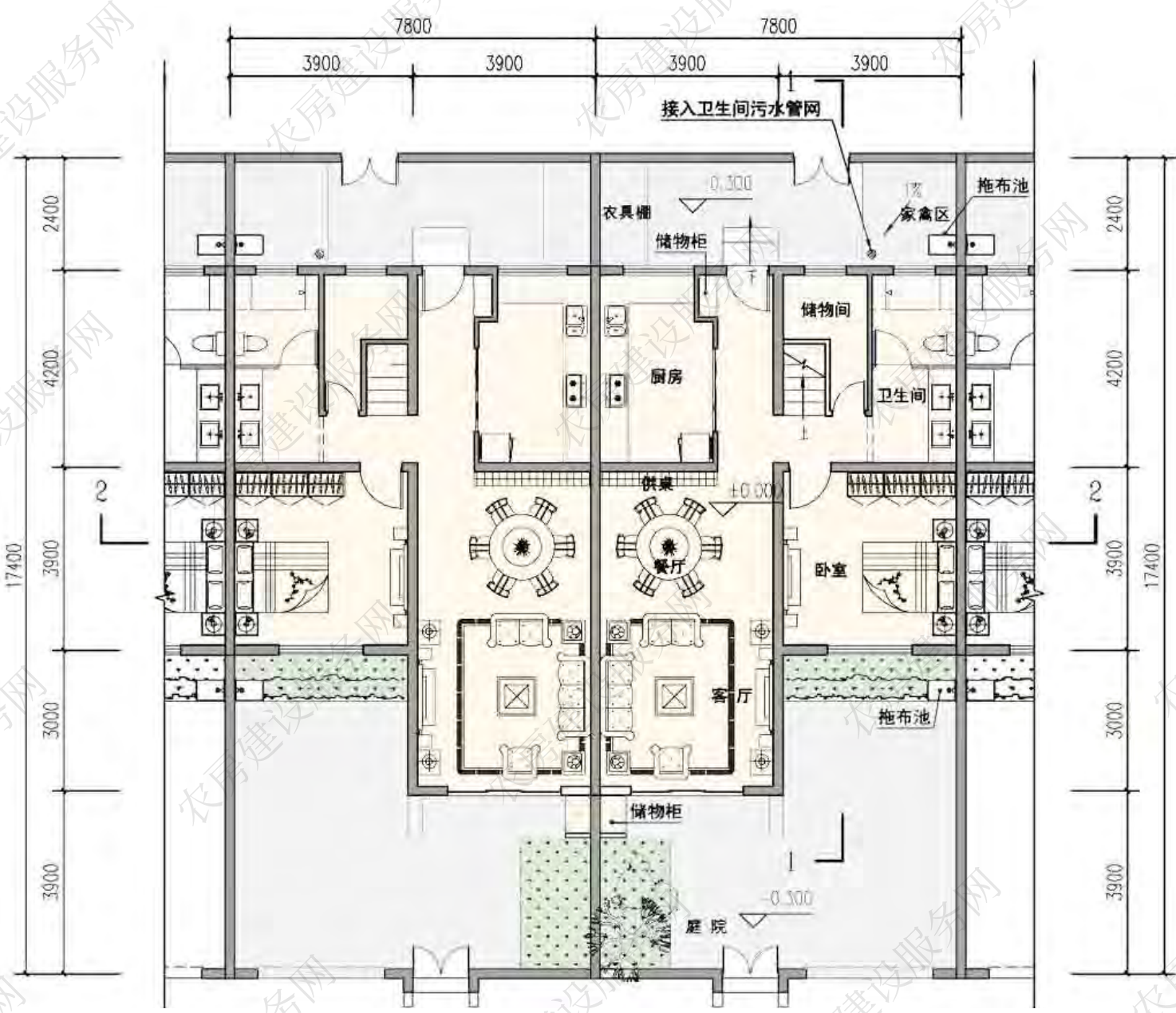
一层平面图
