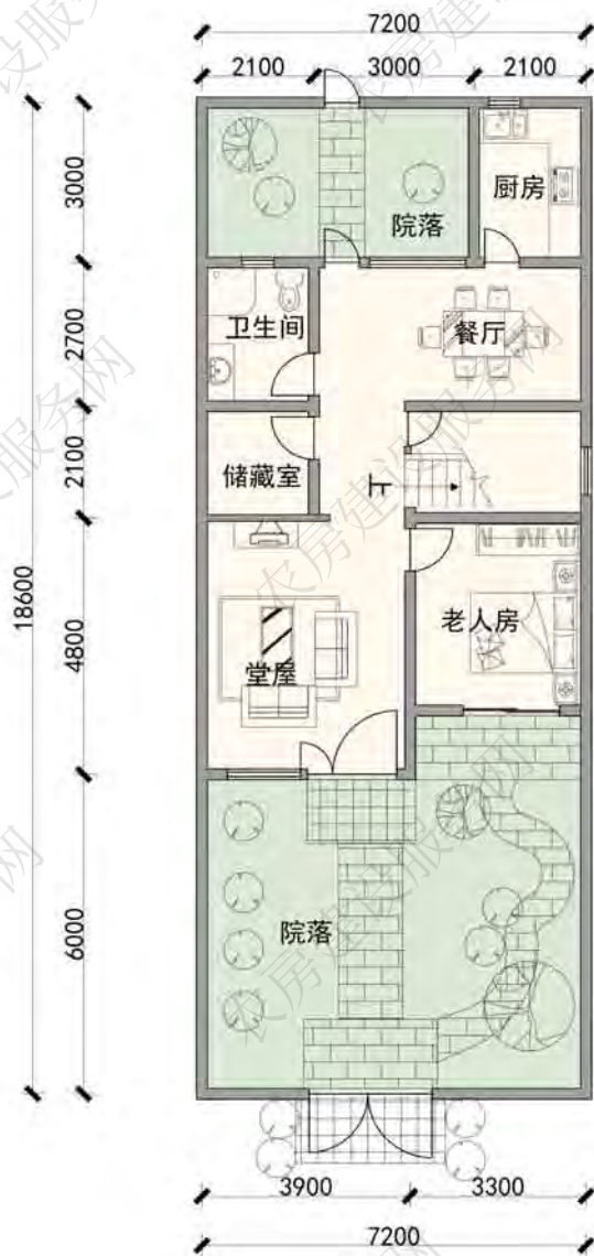
一层平面图
