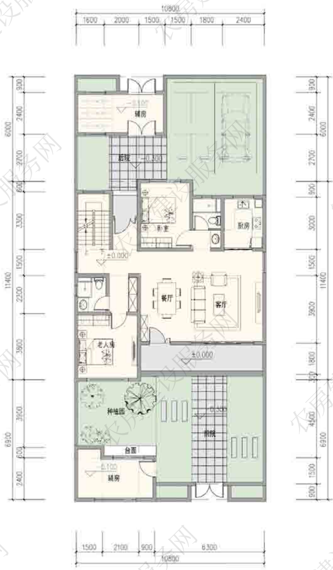
一层平面图
