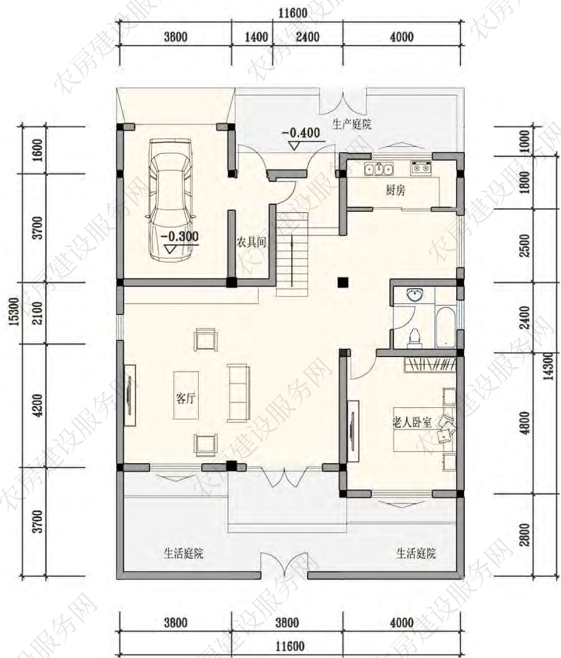
一层平面图
