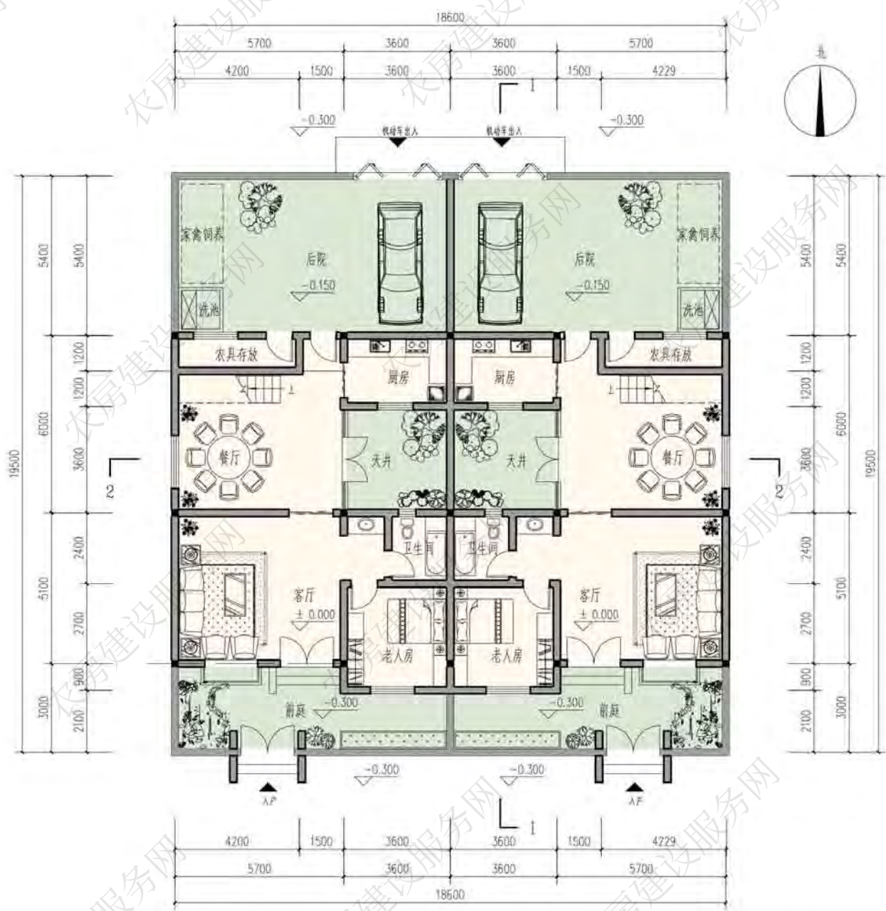
一层平面图
