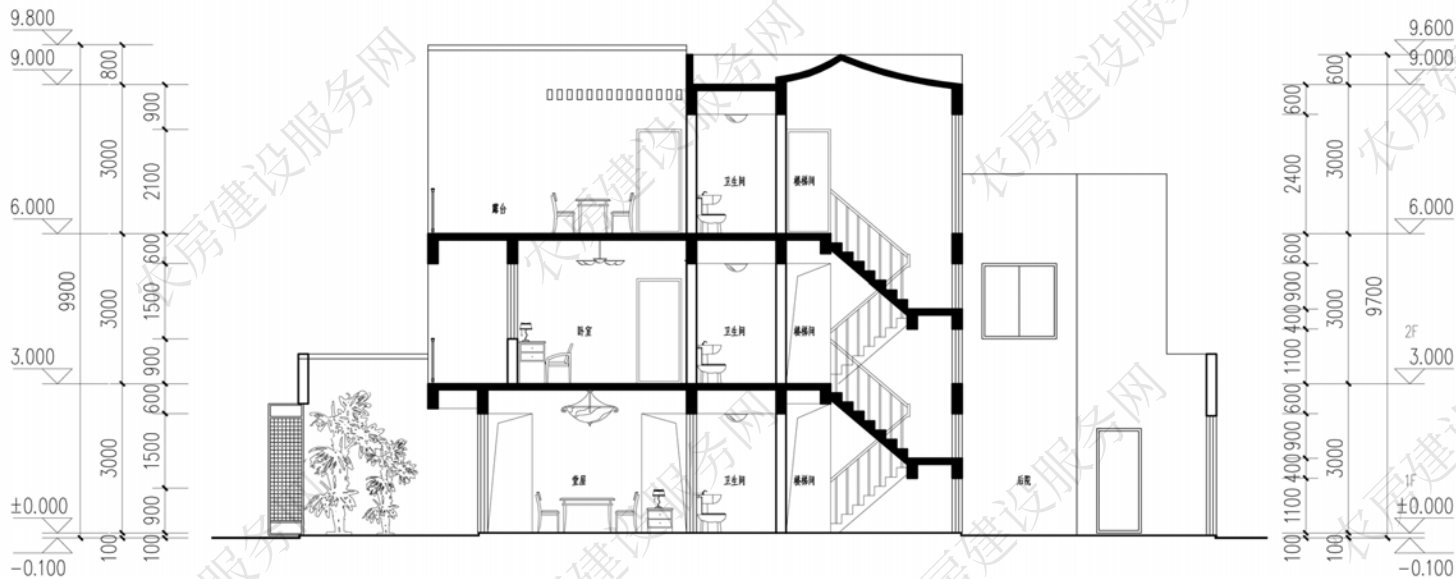
2-2 剖面图
