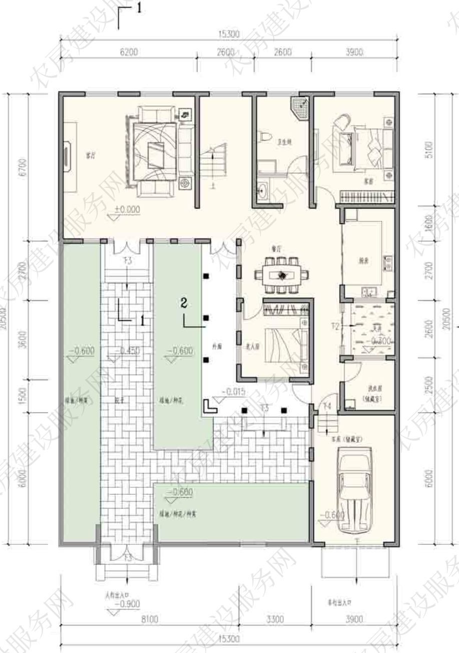
一层平面图
