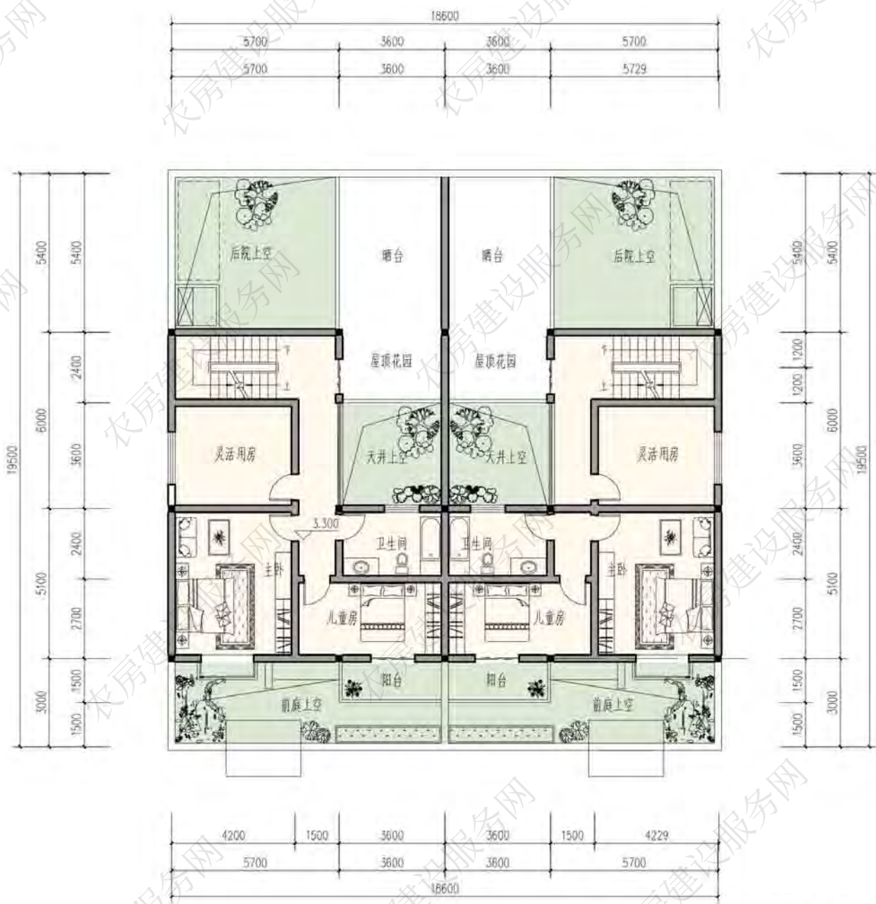
二层平面图
