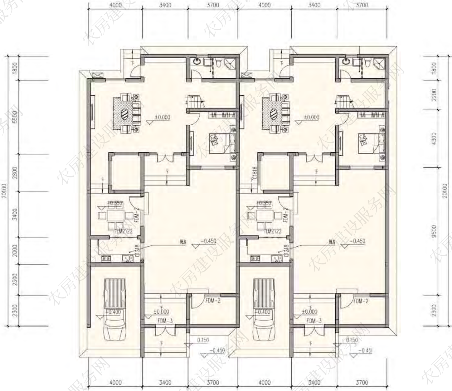
一层平面图
