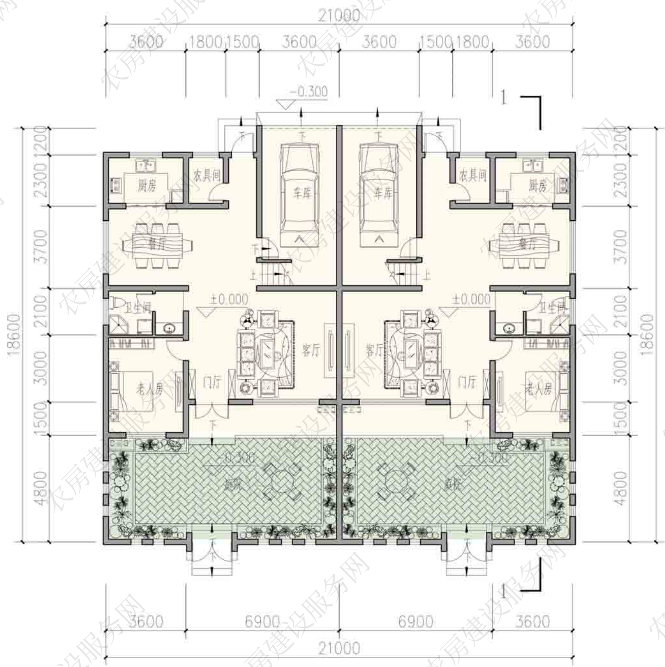
一层平面图
