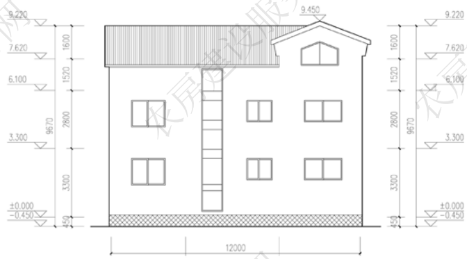
北立面图
