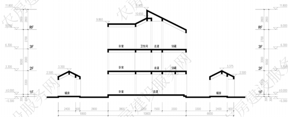
1-1 剖面图
