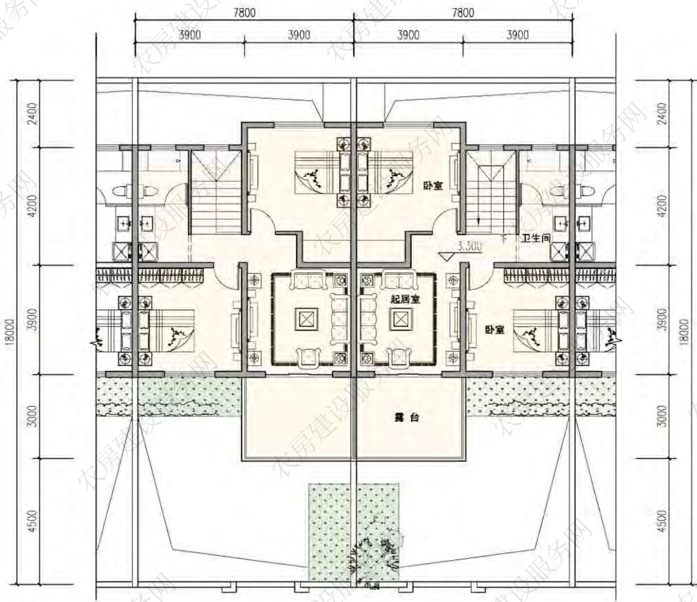
二层平面图
