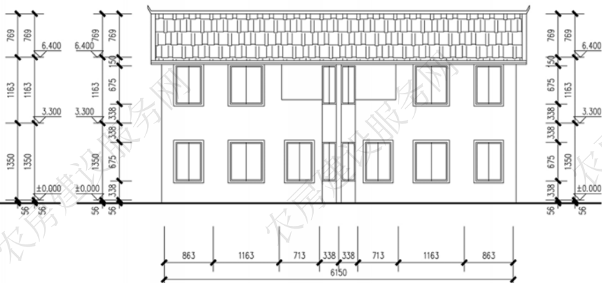
北立面图
