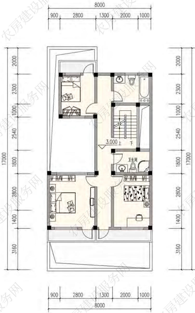
二层平面图
