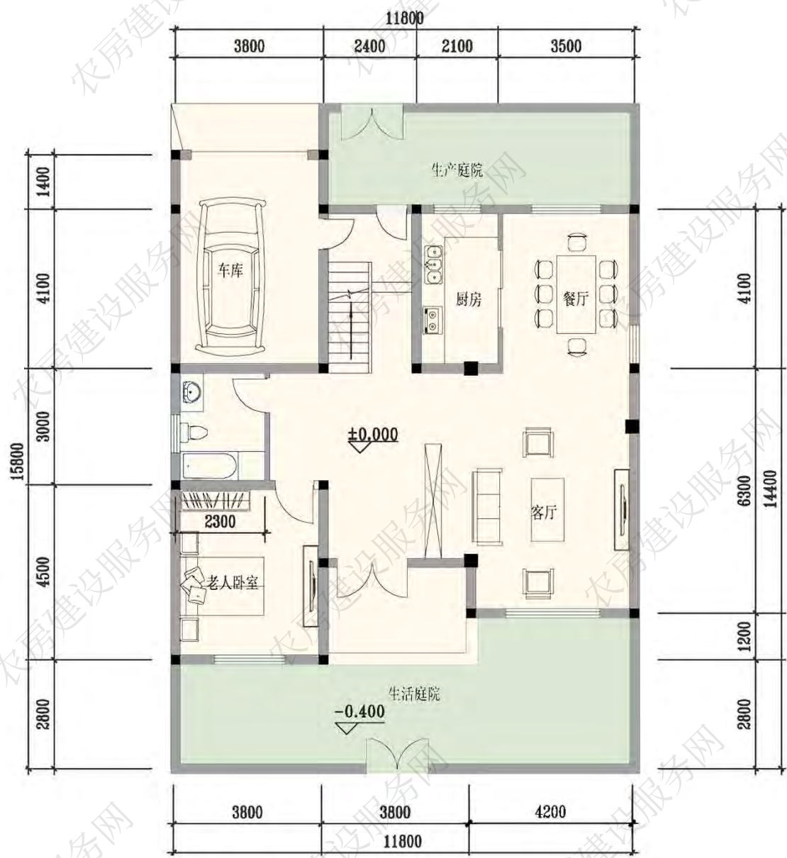
一层平面图
