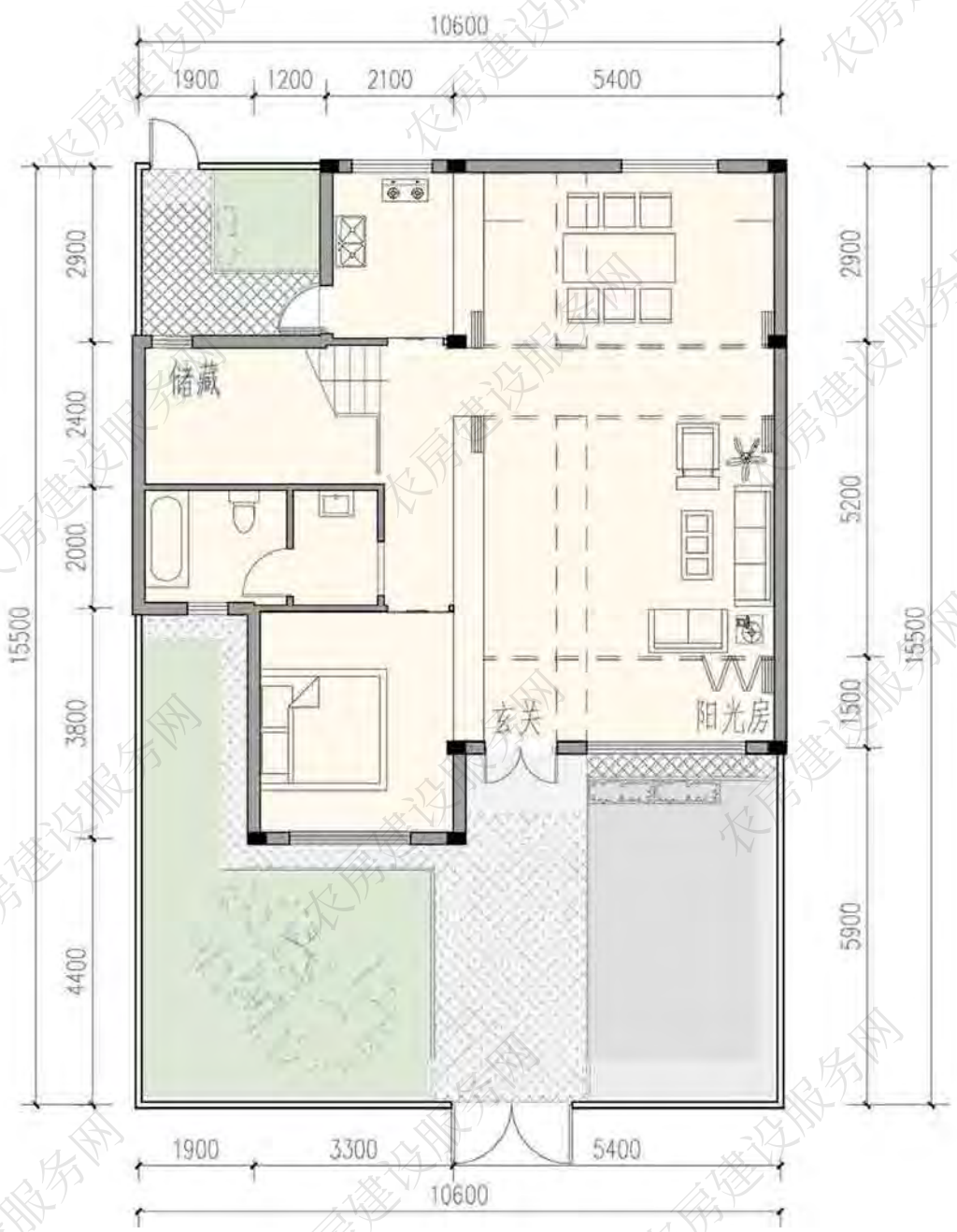
一层平面图
