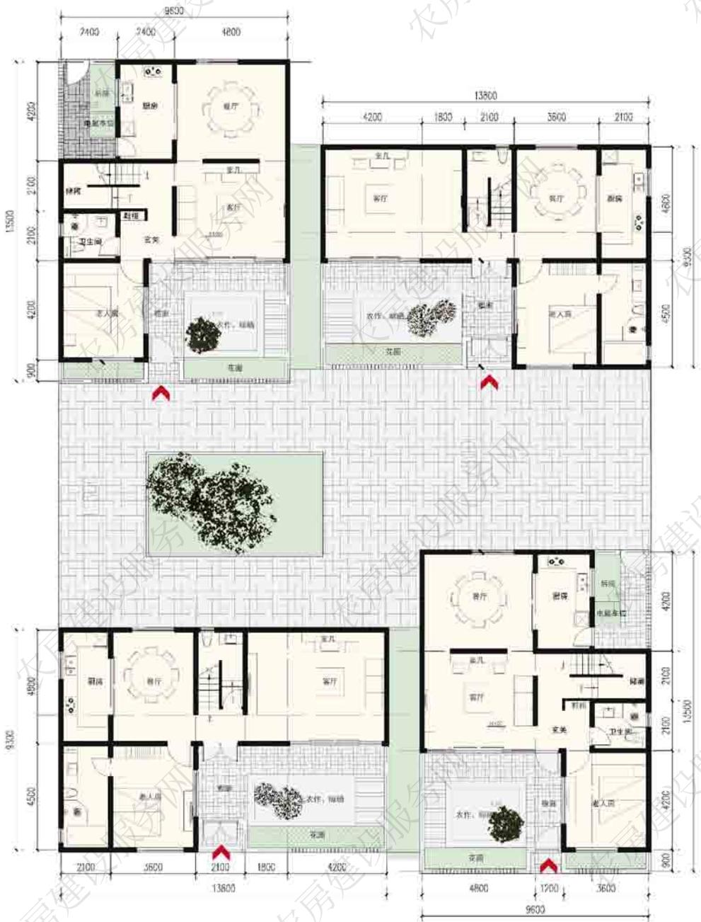
130m 2 宅基地四户组团底层平面
