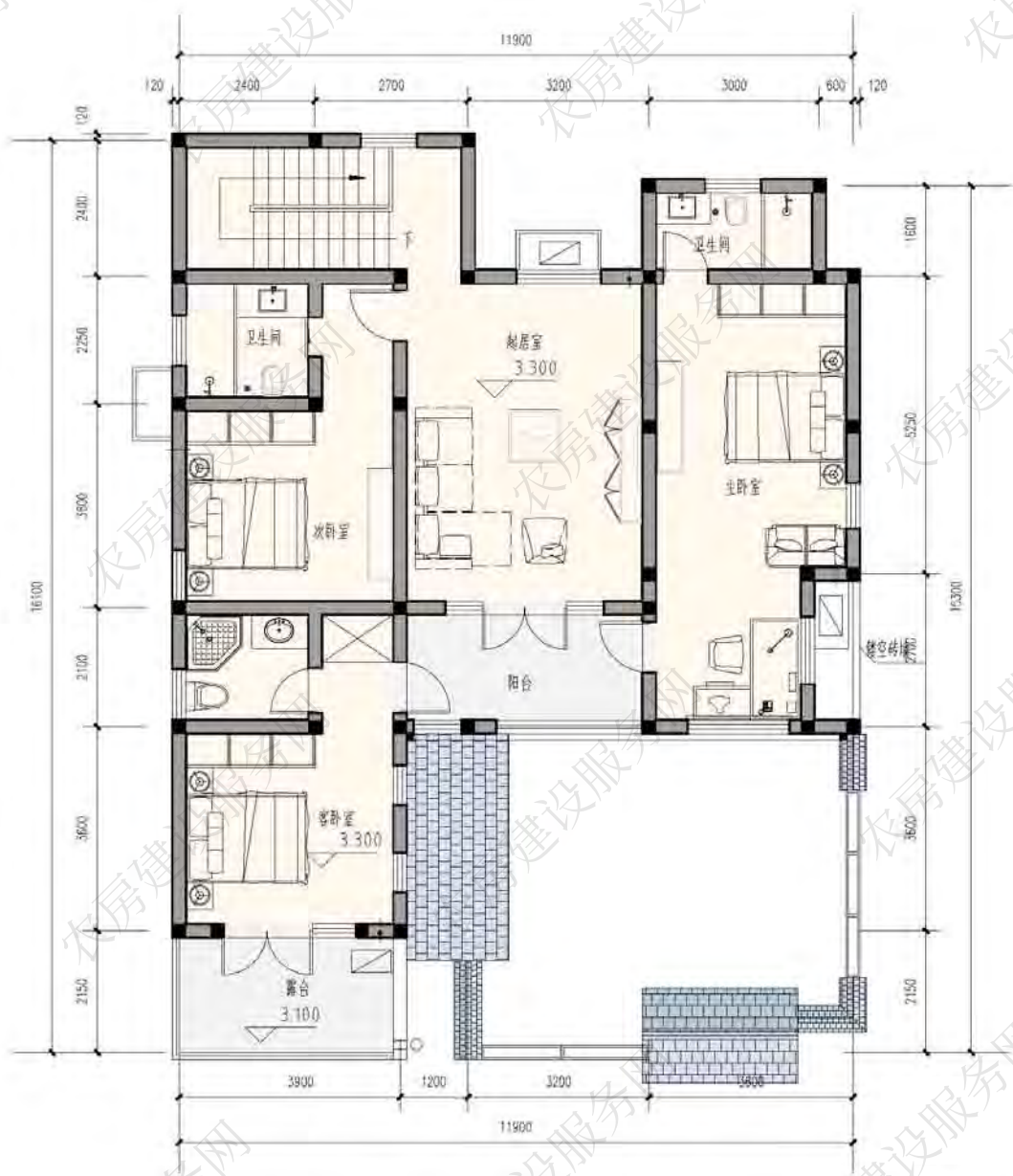
二层平面图
