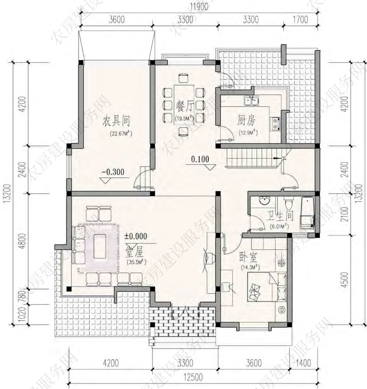
一层平面图
