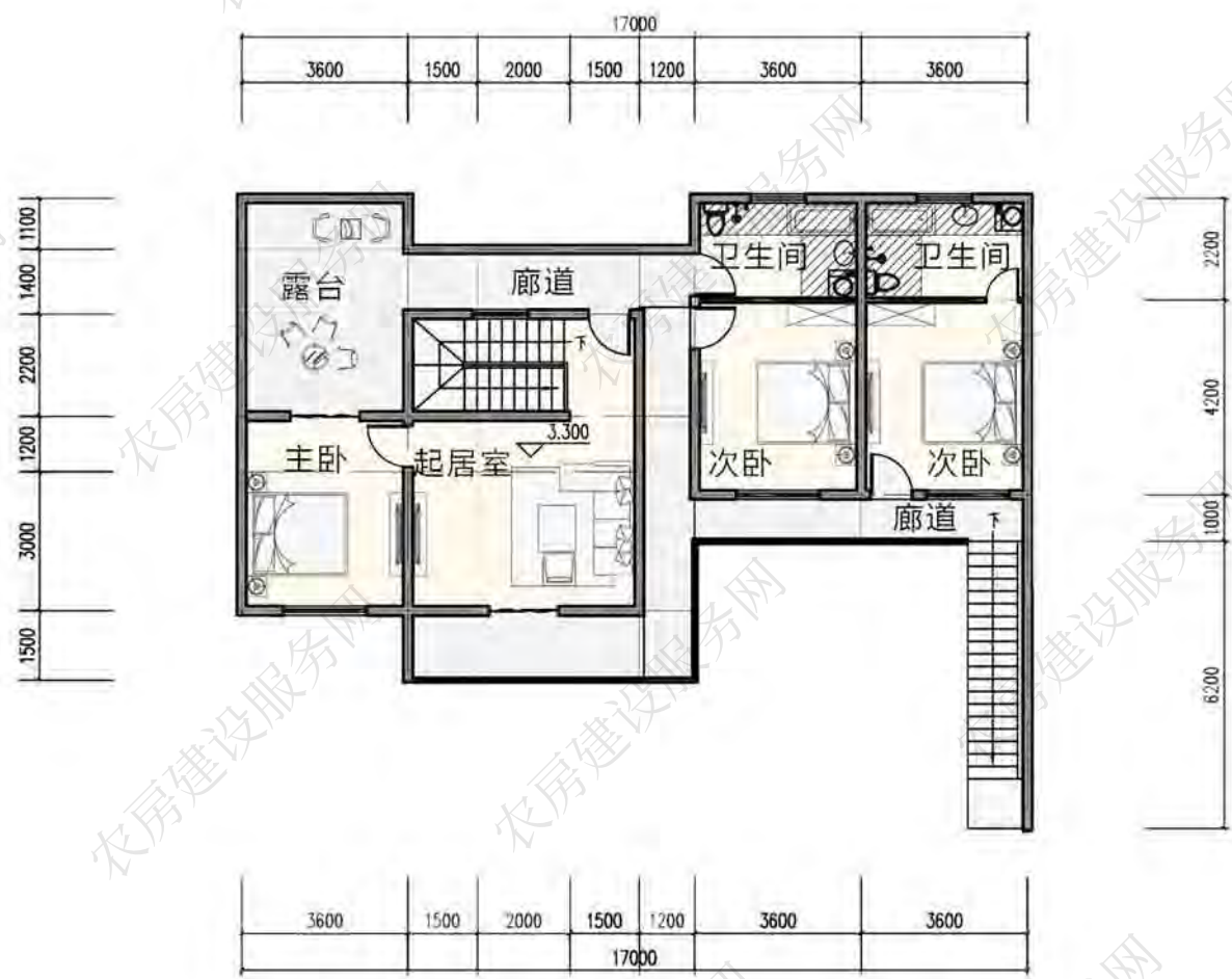
二层平面图
