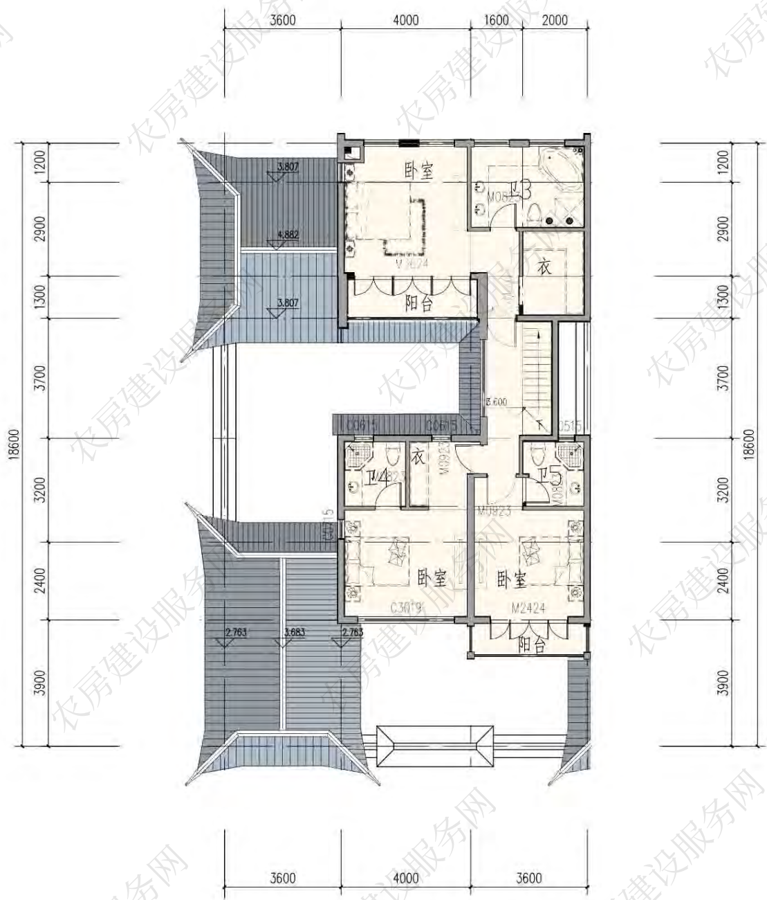
二层平面图
