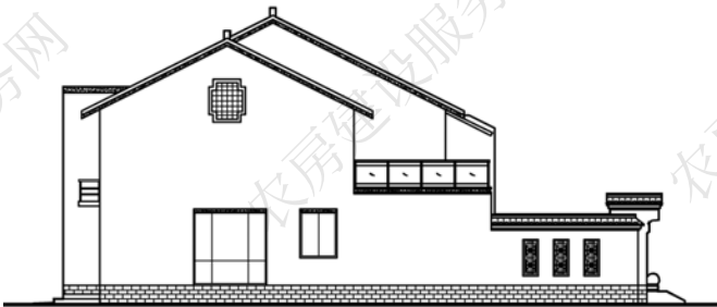
西立面图
