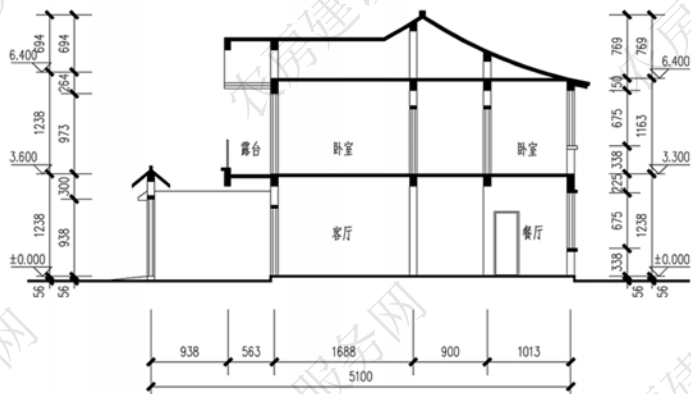
1-1 剖面图
