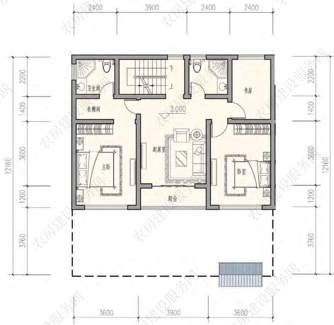
二层平面图
