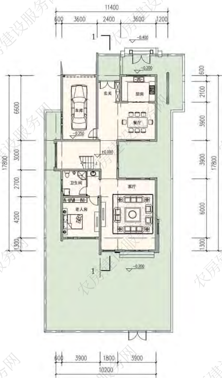
一层平面图
