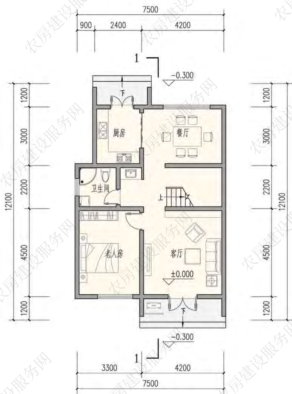
一层平面图
