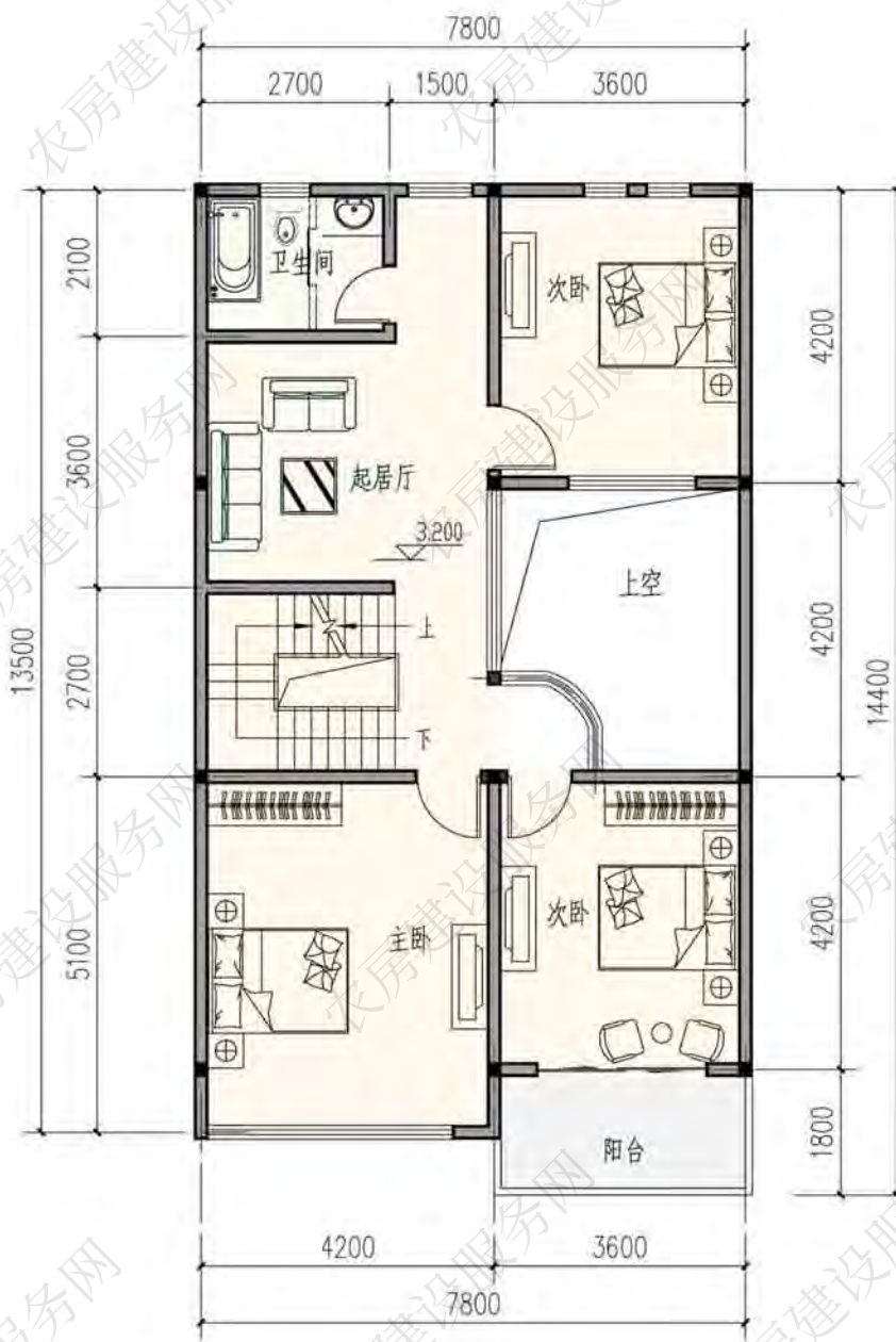
二层平面图
