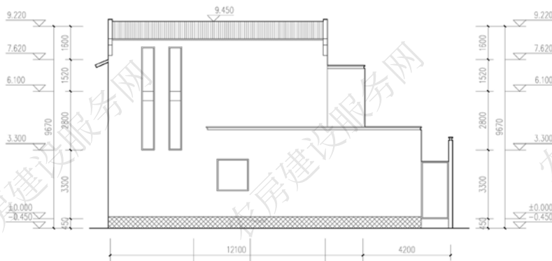
西立面图
