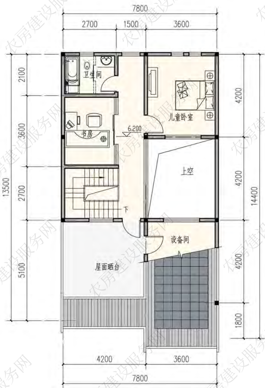
三层平面图
