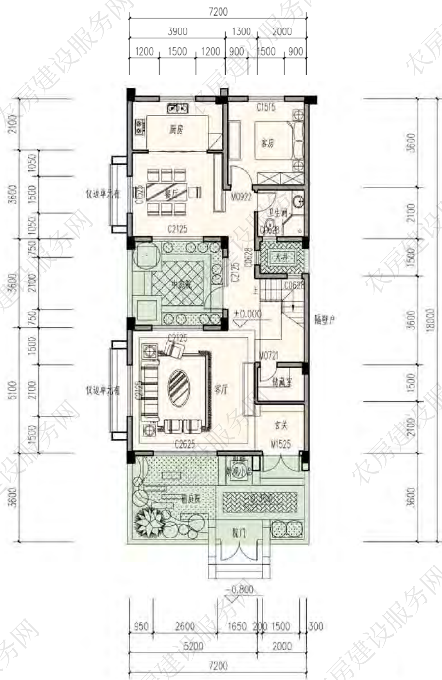
一层平面图
