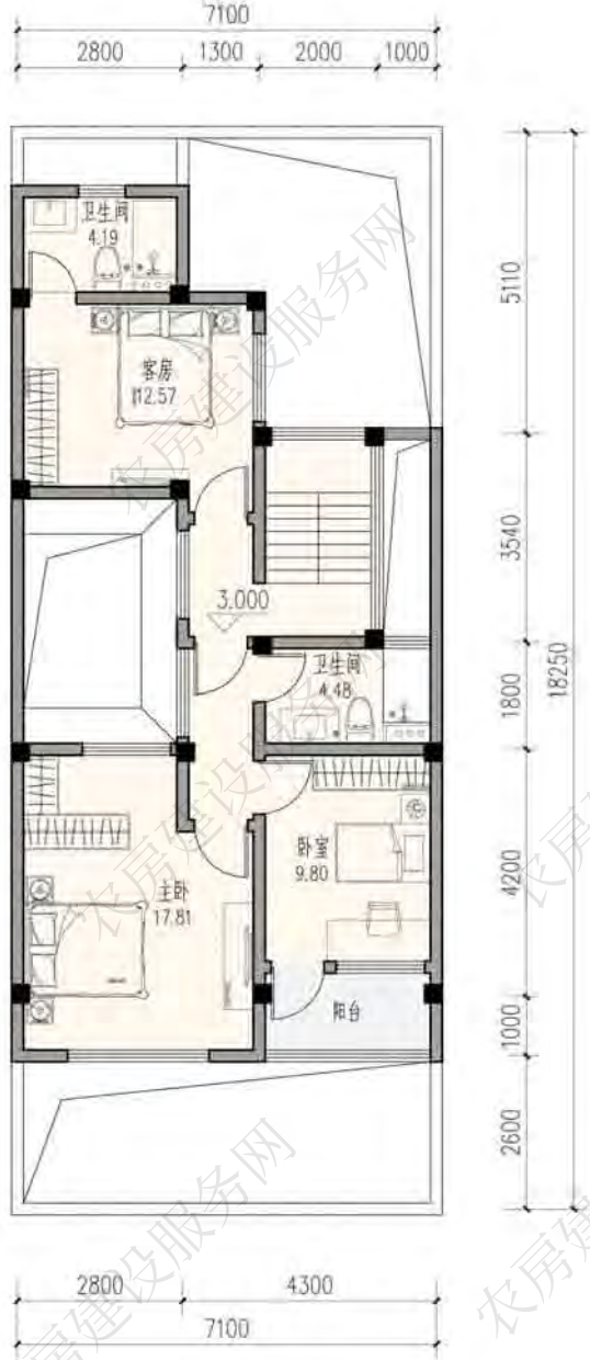
二层平面图
