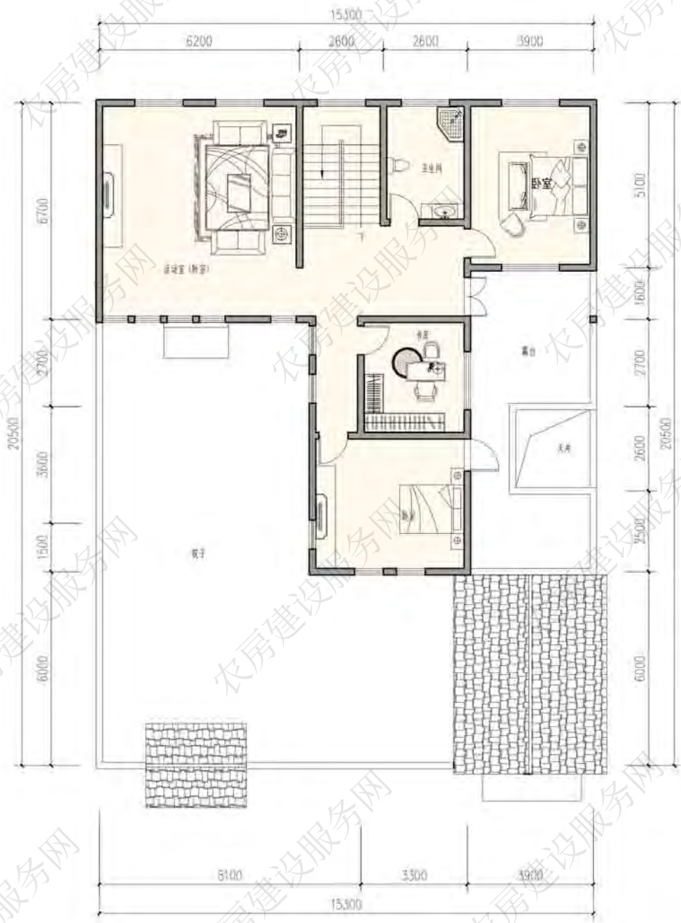
二层平面图
