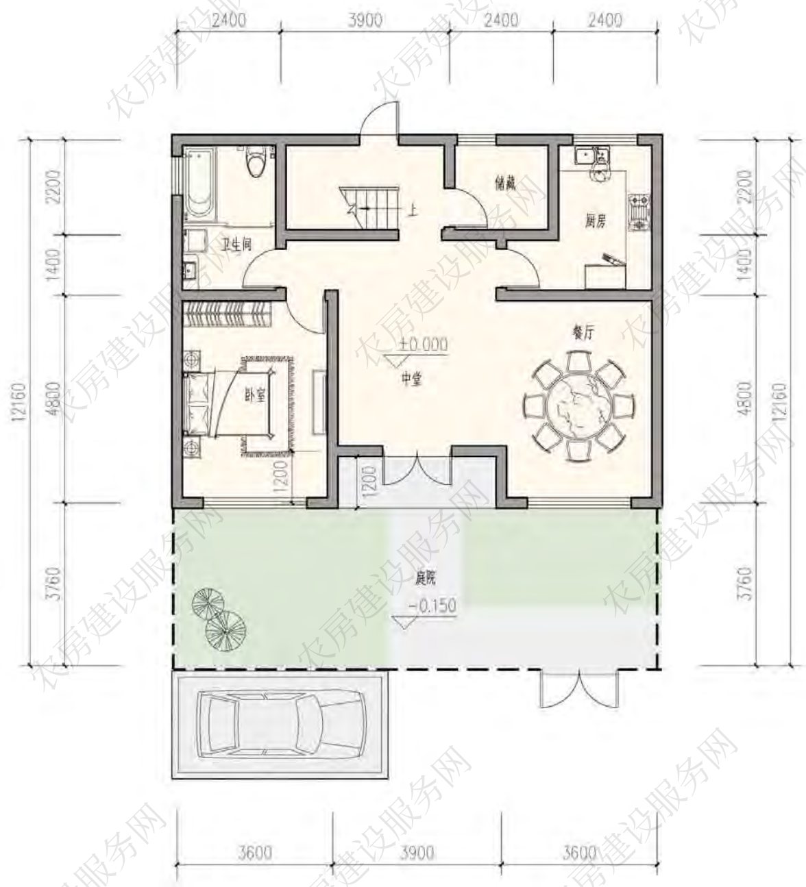
一层平面图
