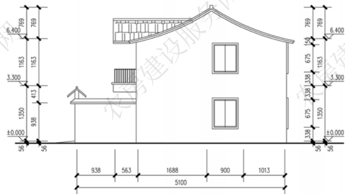
东立面图
