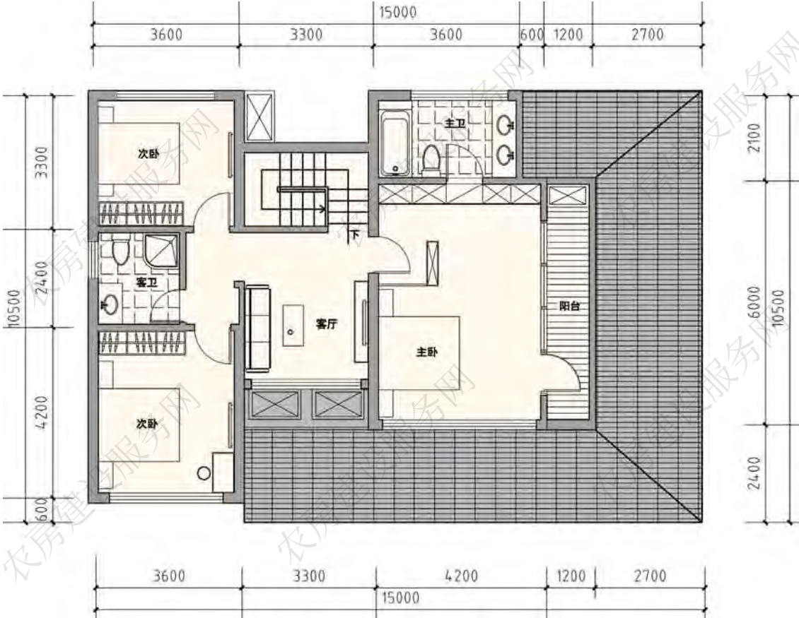
二层平面图
