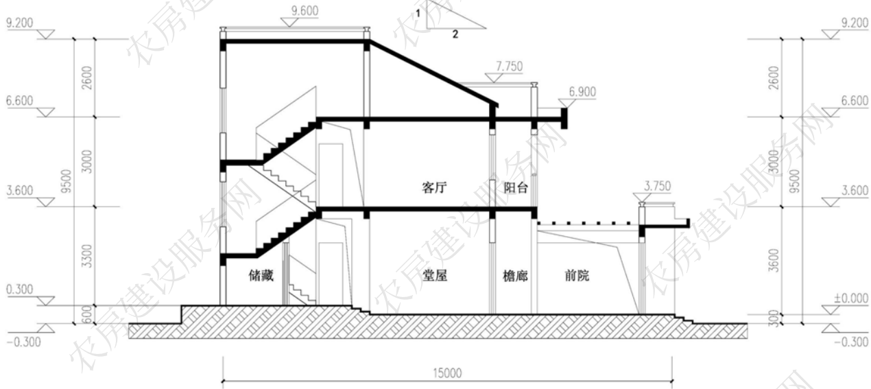
1-1 剖面图
