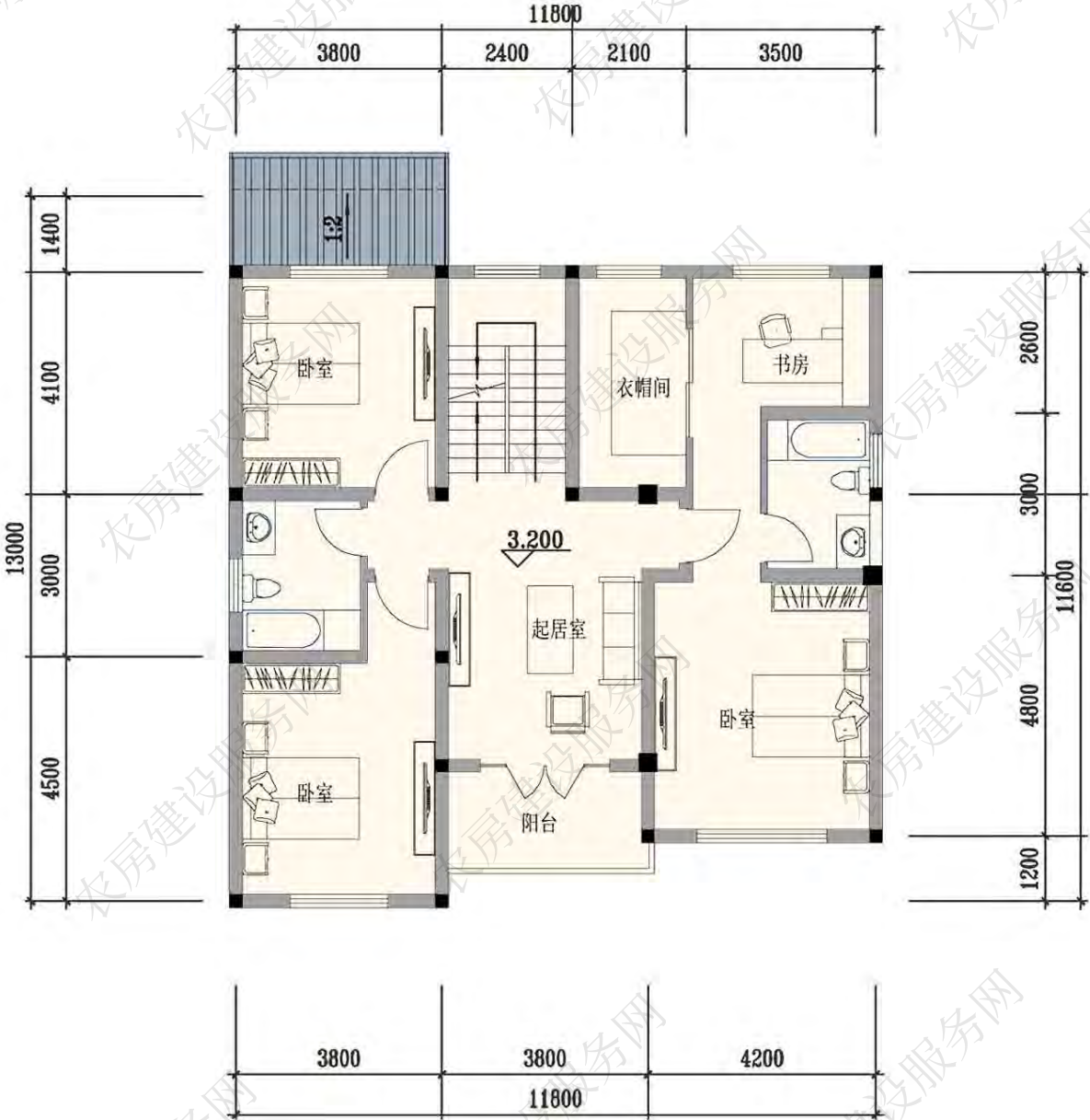
二层平面图
