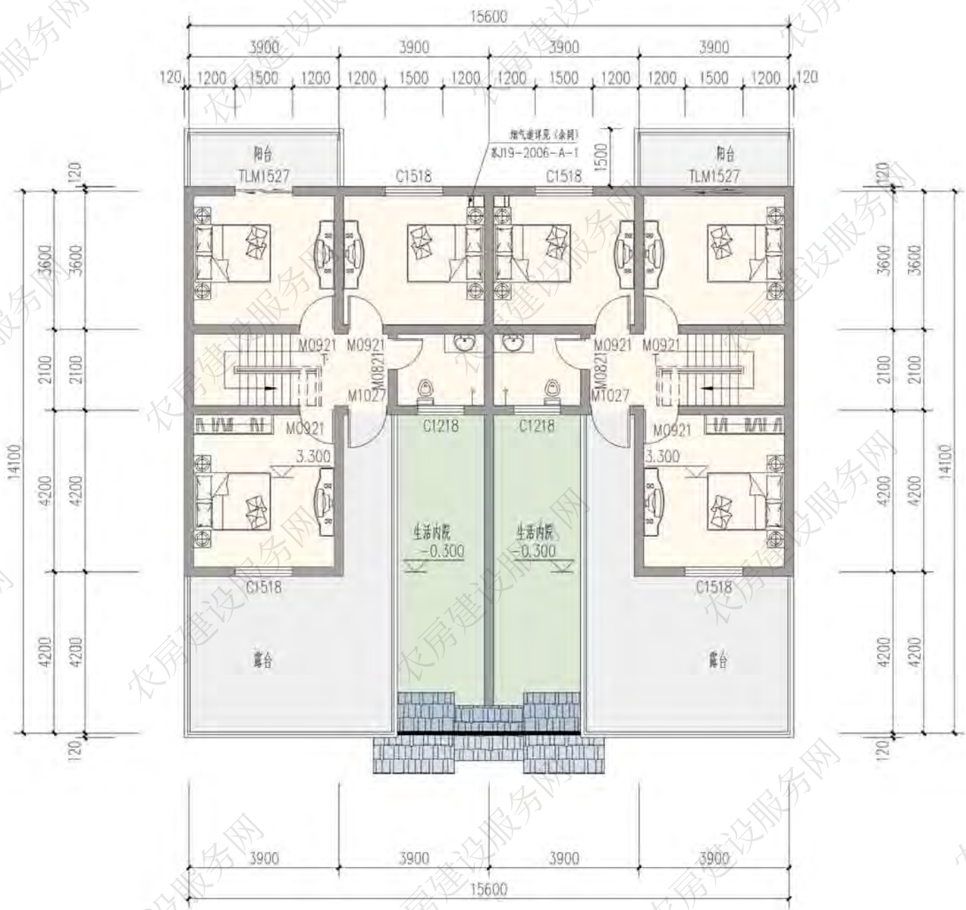
二层平面图
