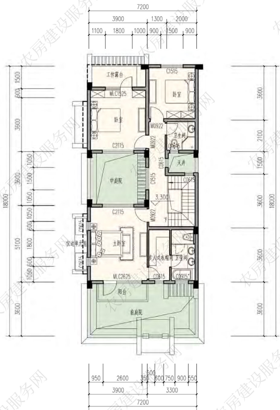
二层平面图
