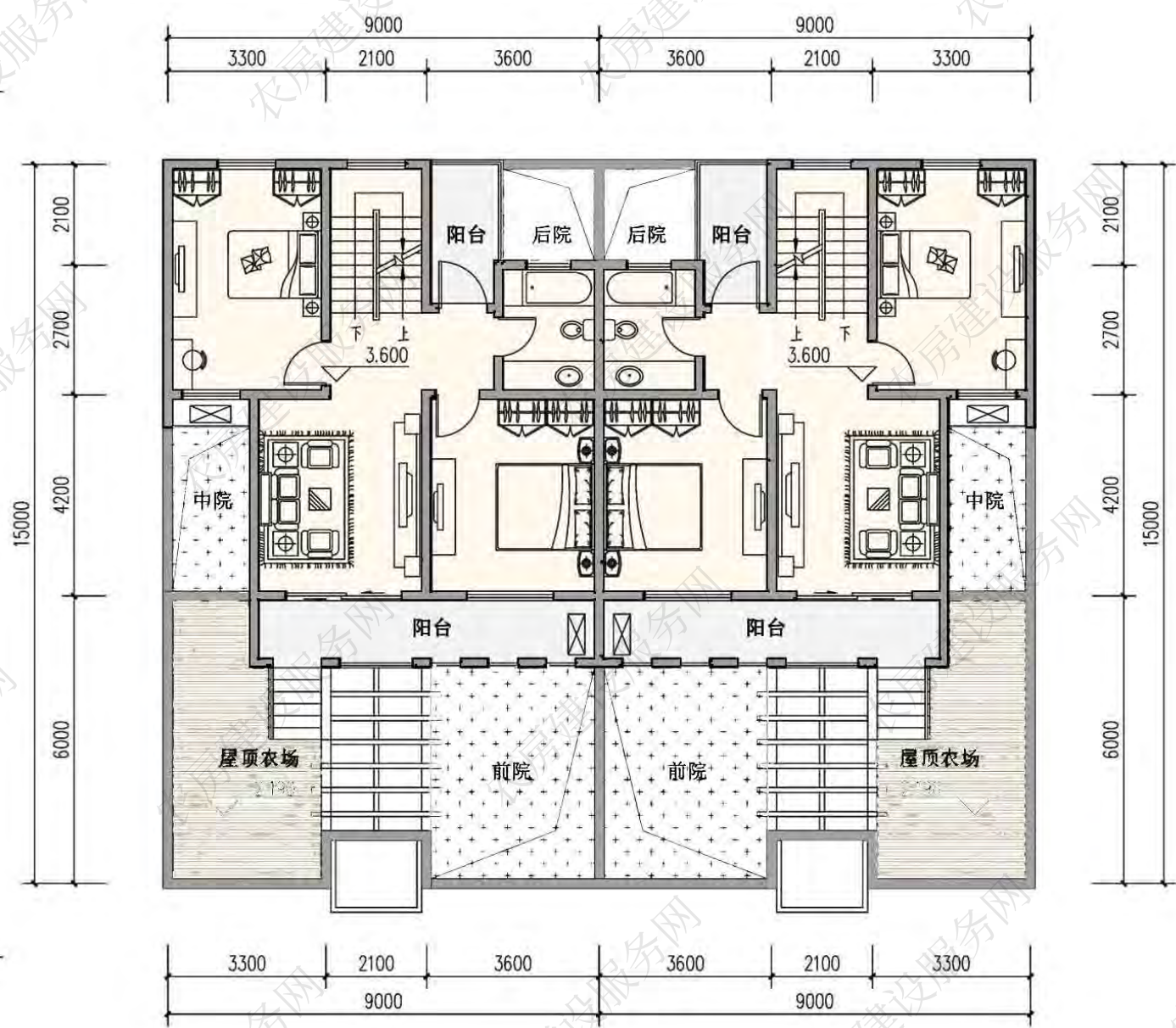
二层平面图
