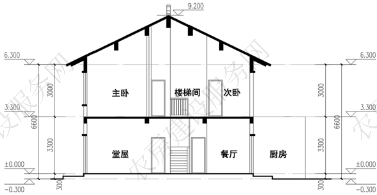
剖面图
