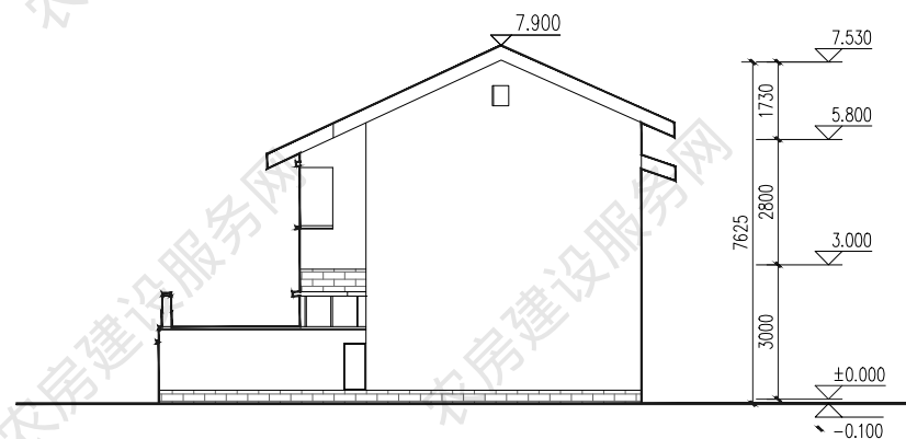
东立面图
