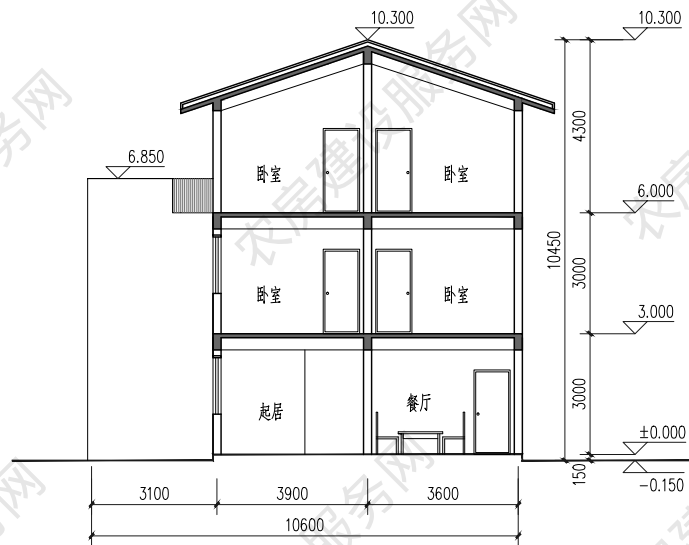
1-1 剖面图
