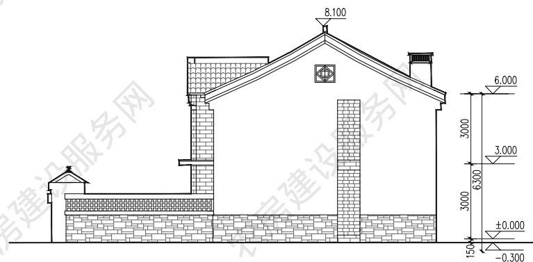
东立面图
