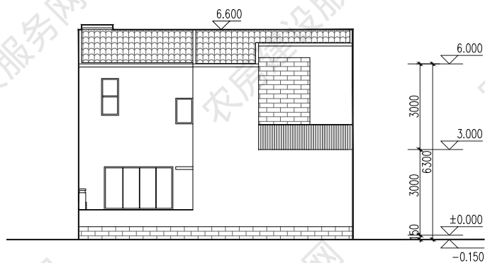
西立面图
