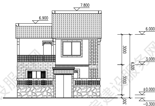
南立面图
