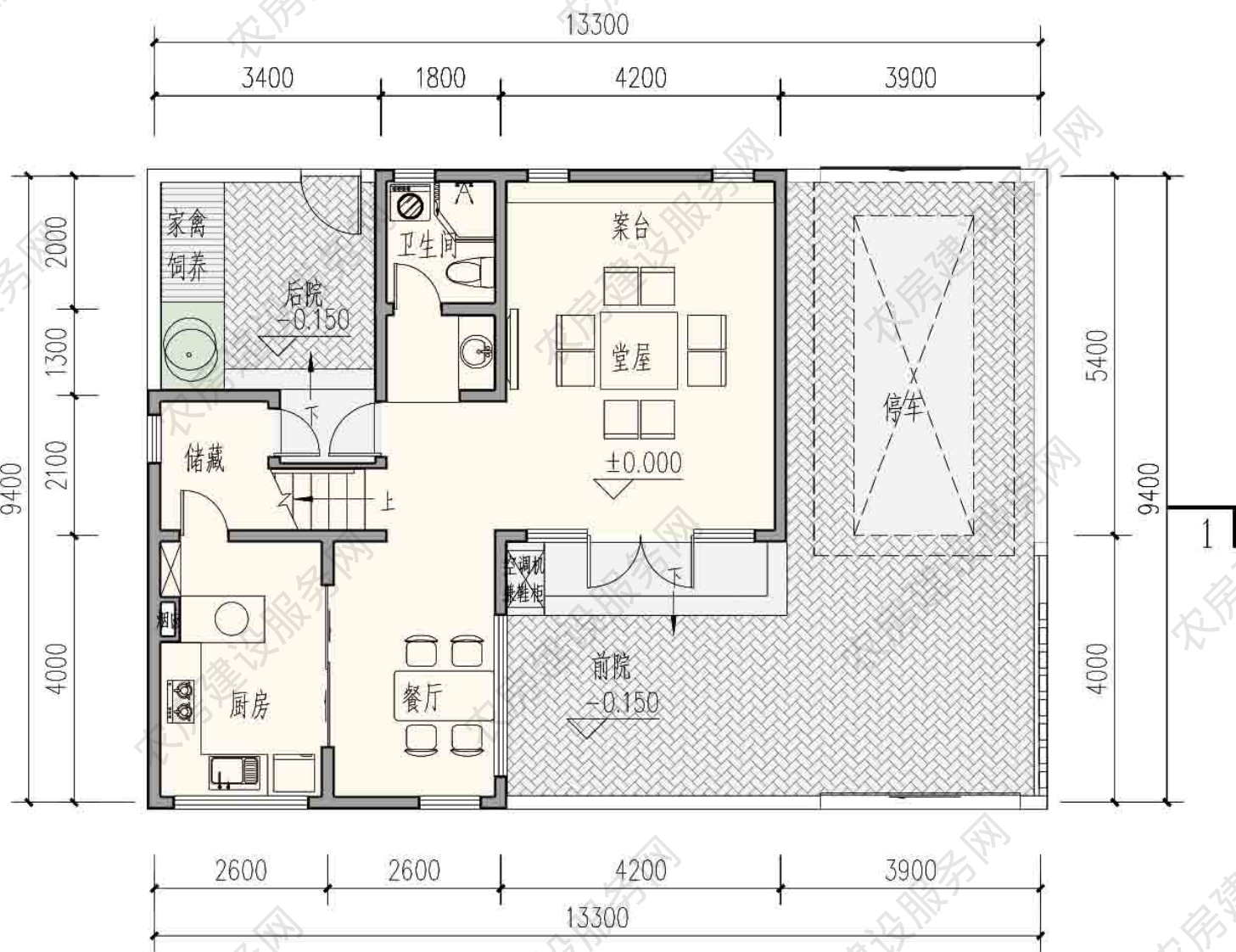
一层平面图
