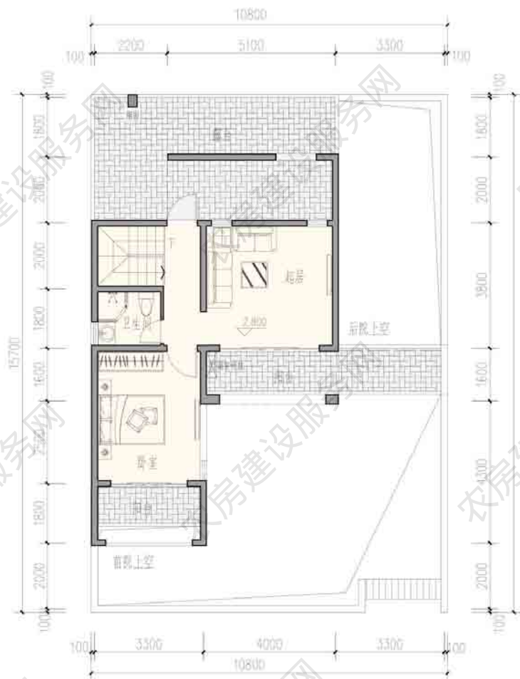
二层平面图 本层建筑面积 44 平方米
