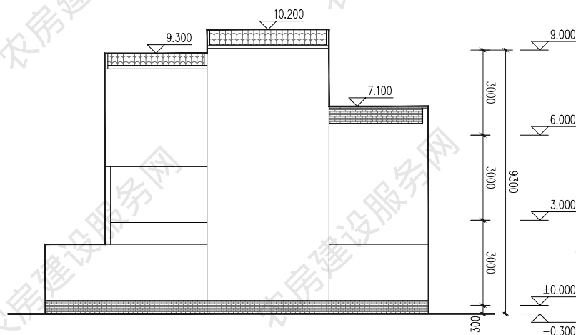
东立面图
