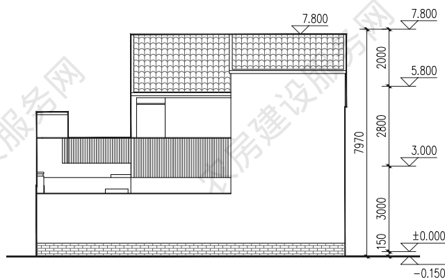
东立面图
