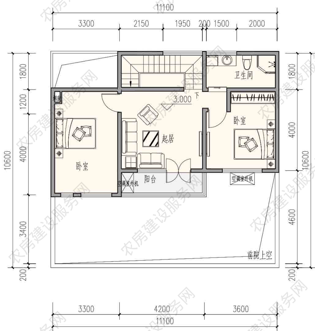
二层平面图
