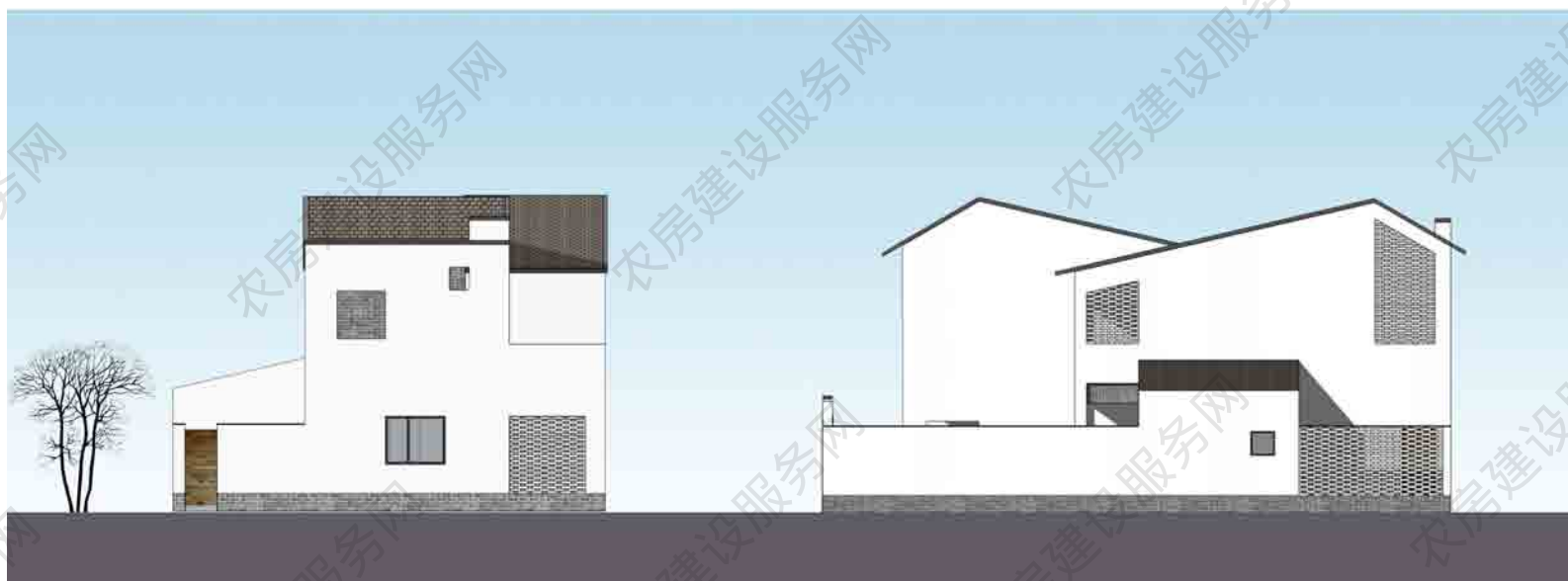
北立面图
