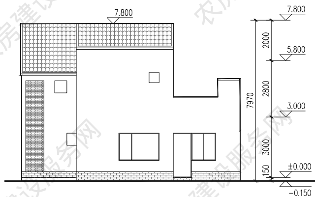
西立面图
