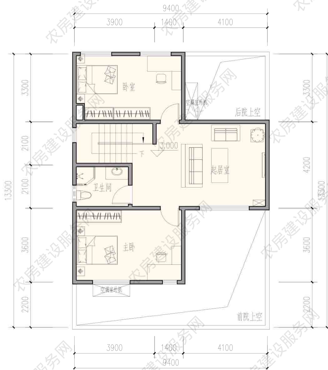
二层平面图
