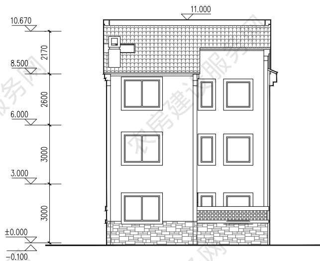
北立面图
