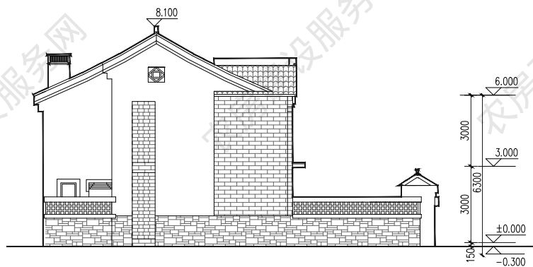
西立面图
