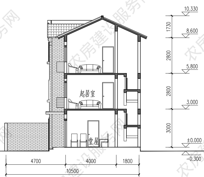
1-1 剖面图
