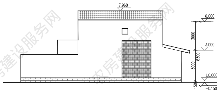
东立面图
