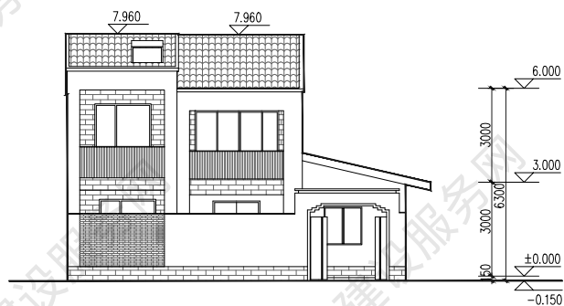
南立面图
