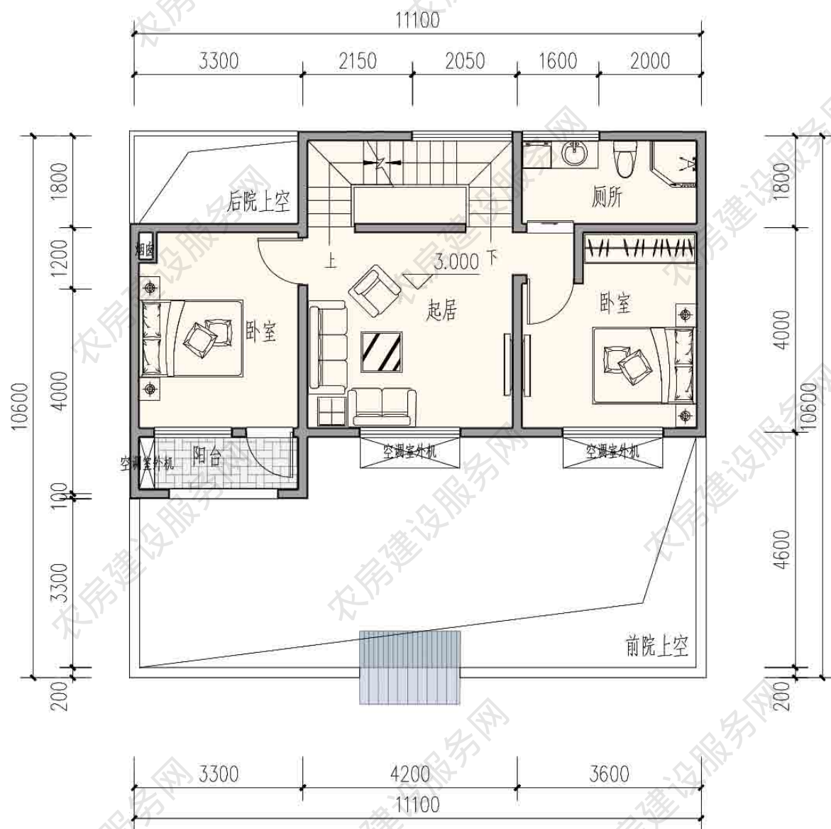
二层平面图
