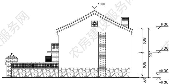
东立面图
