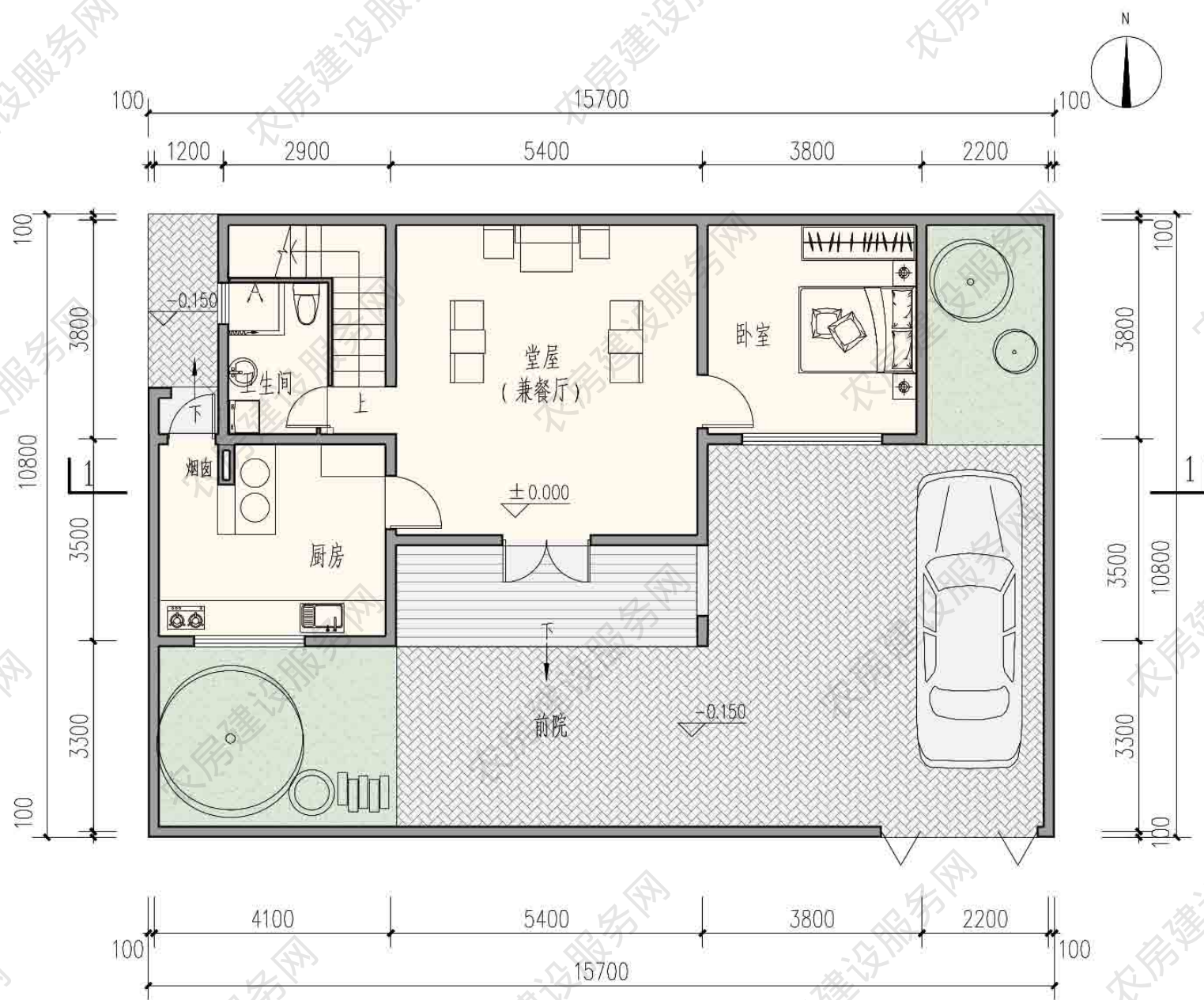
一层平面图
