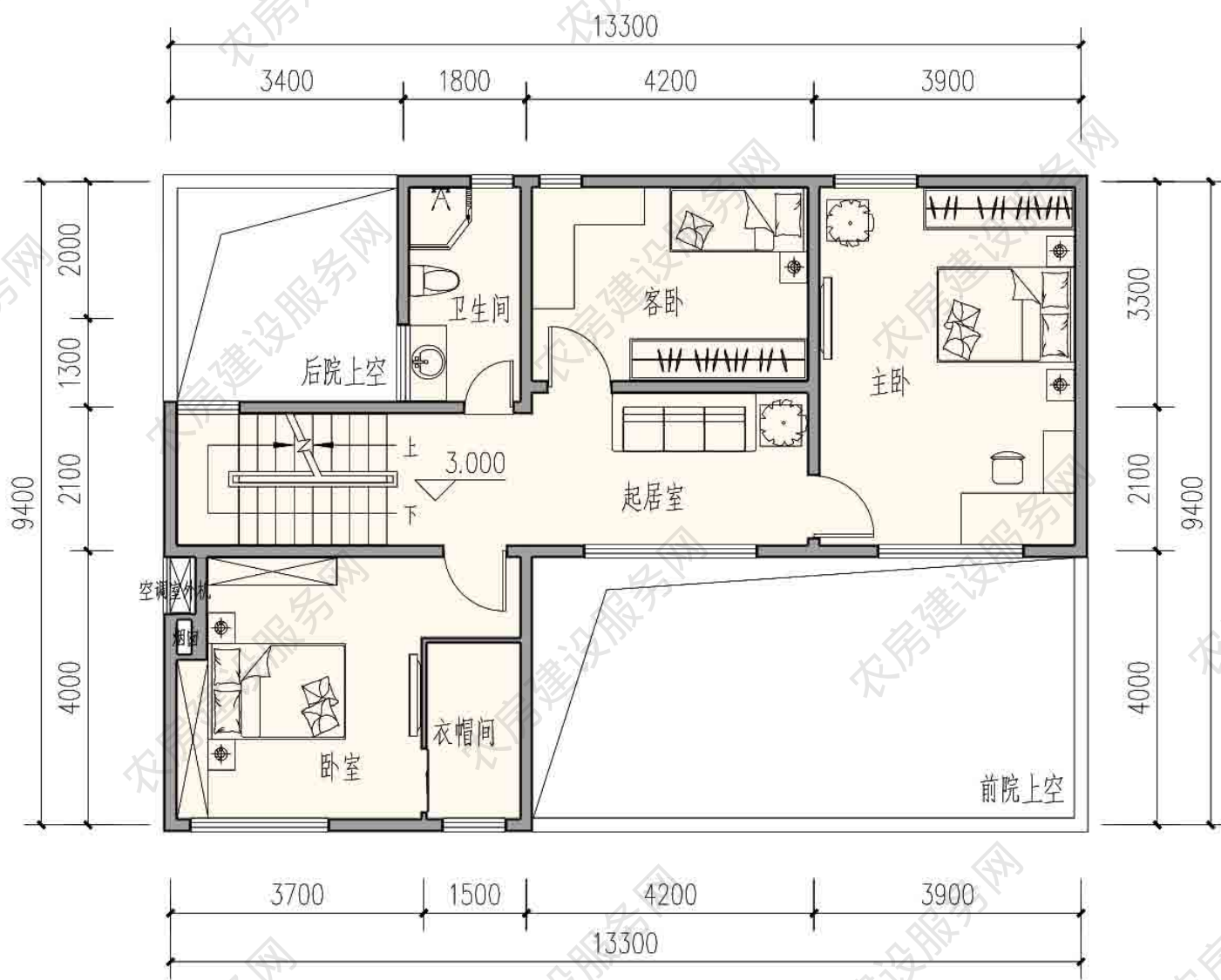
二层平面图
