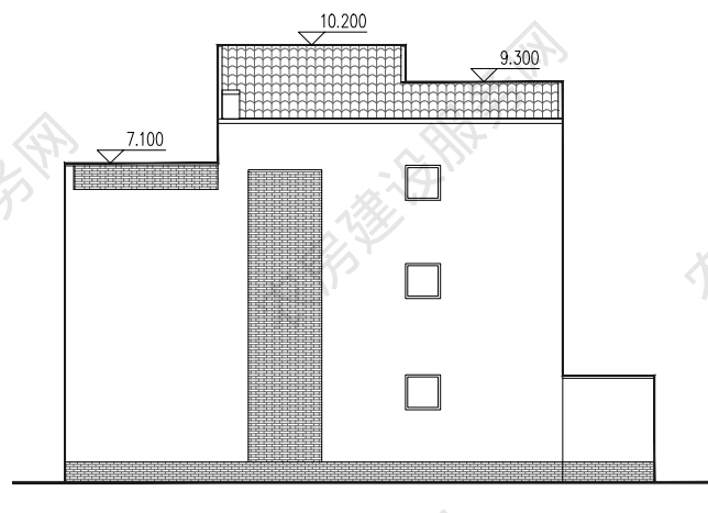
西立面图
