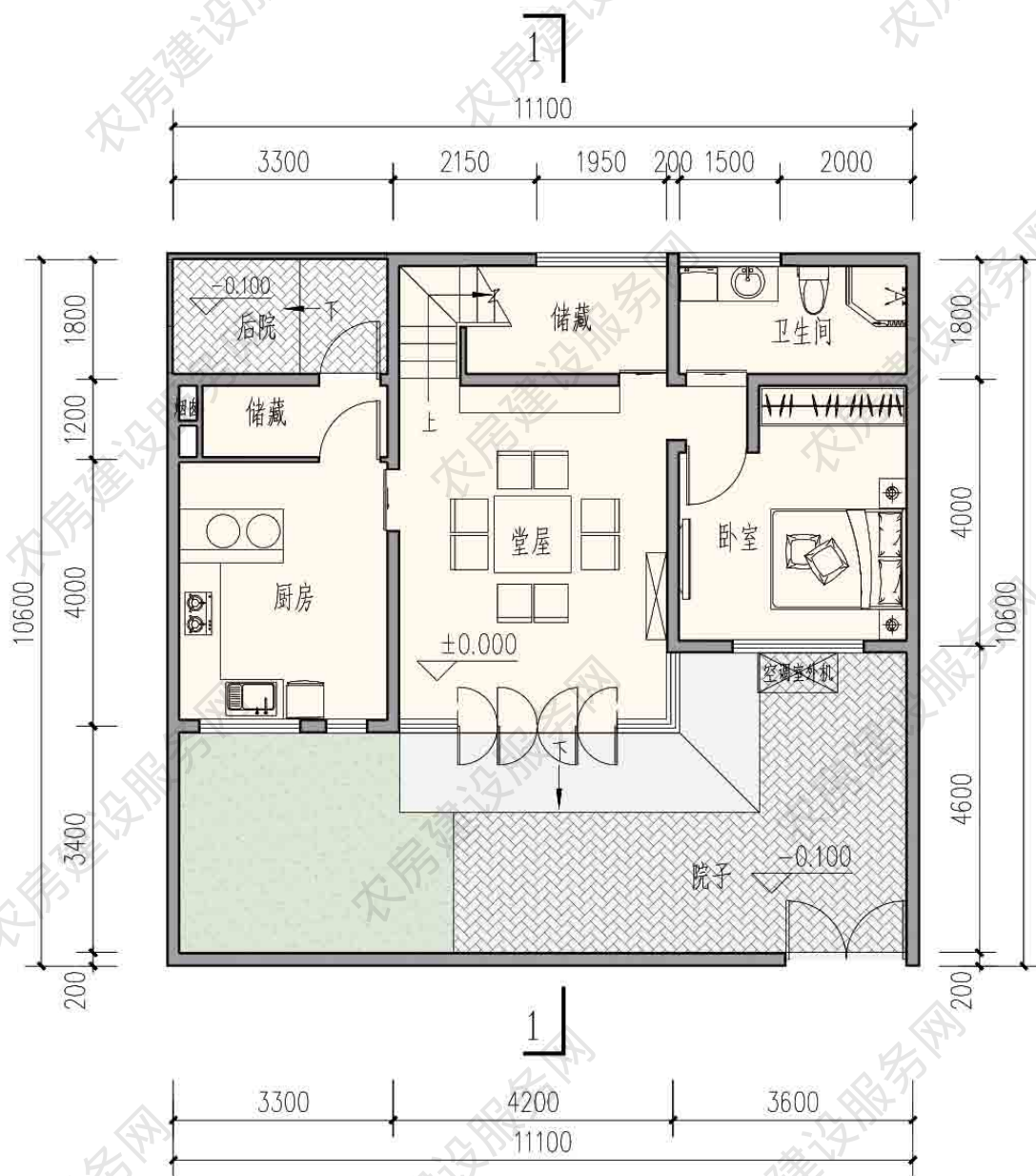
一层平面图 本层建筑面积 66 平方米
