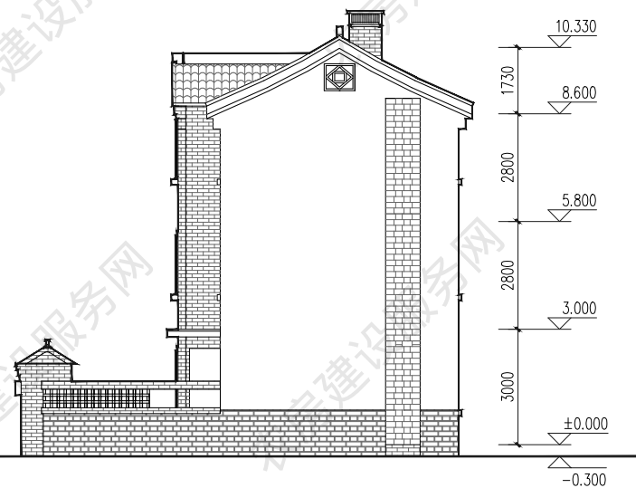
东立面图
