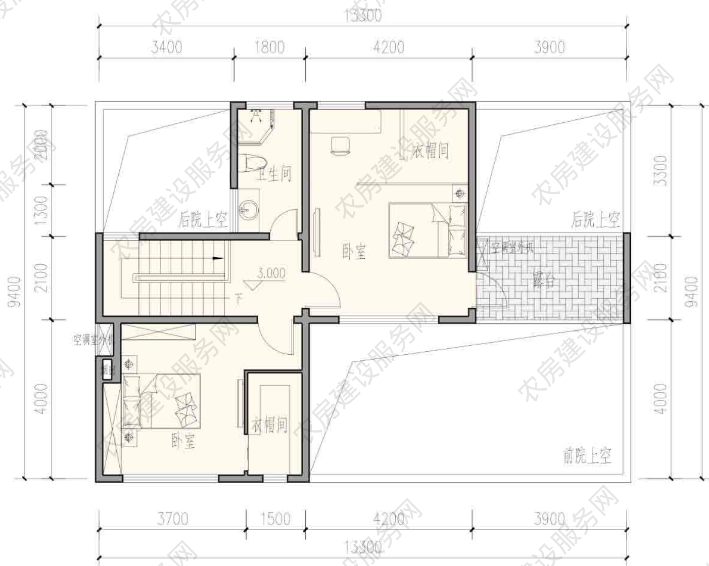
二层平面图
