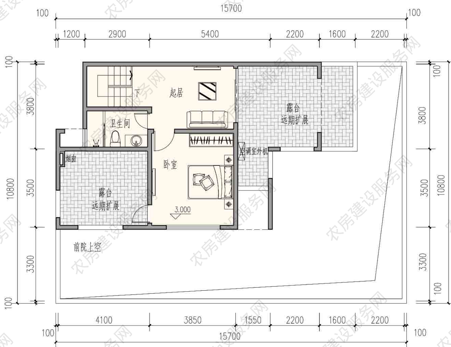
二层平面图
