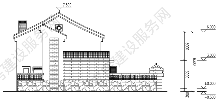
西立面图
