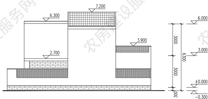
东立面图
