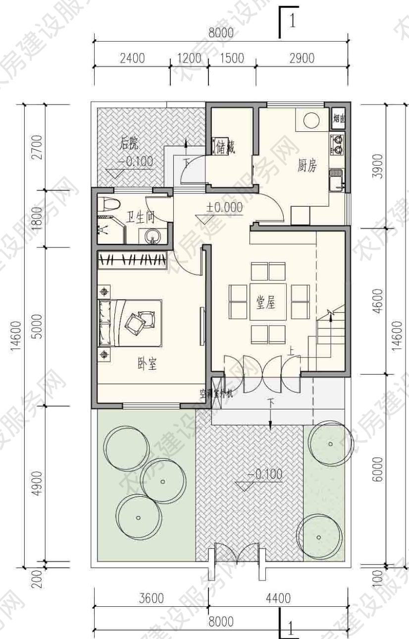
一层平面图 本层建筑面积 65 平方米
