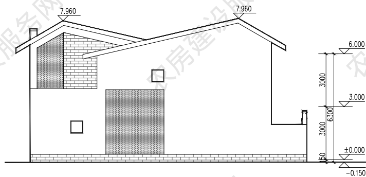
西立面图
