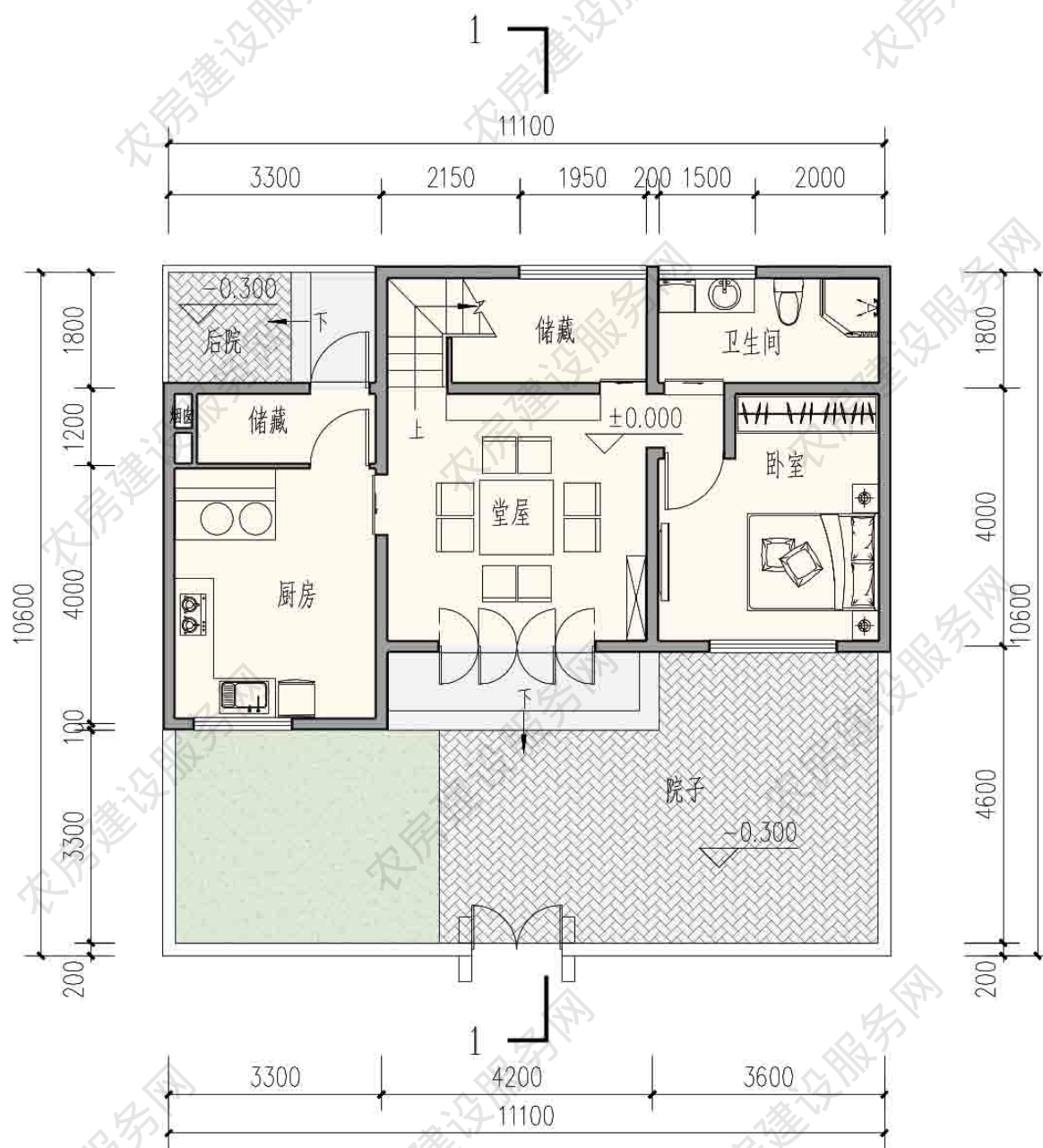
一层平面图 本层建筑面积 66 平方米
