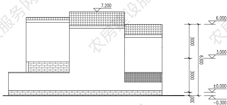
东立面图
