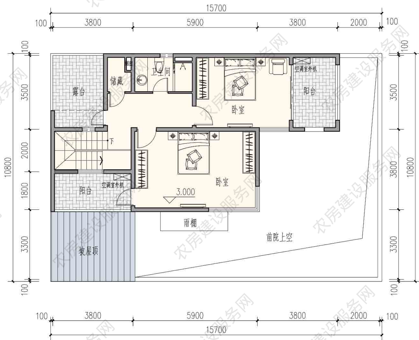
二层平面图
