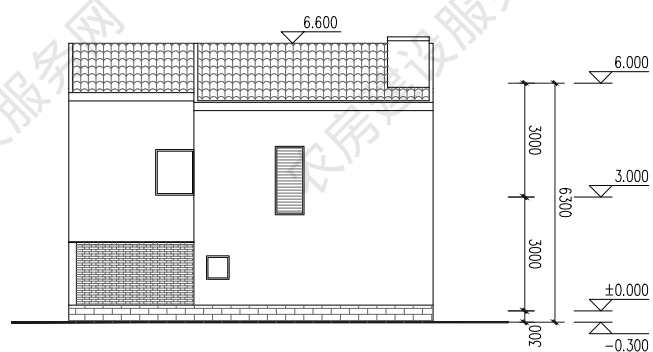
西立面图
