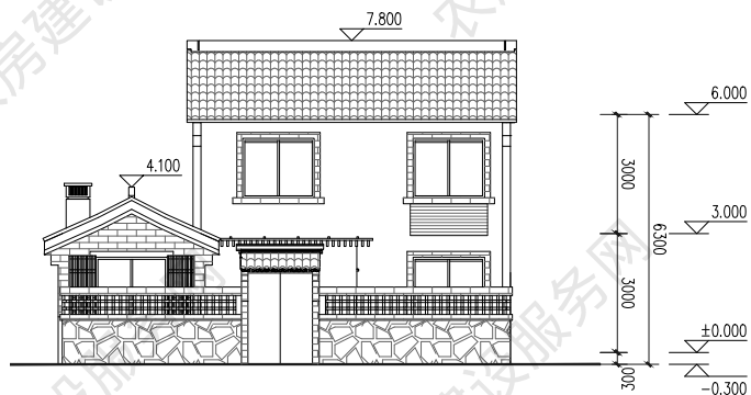
南立面图
