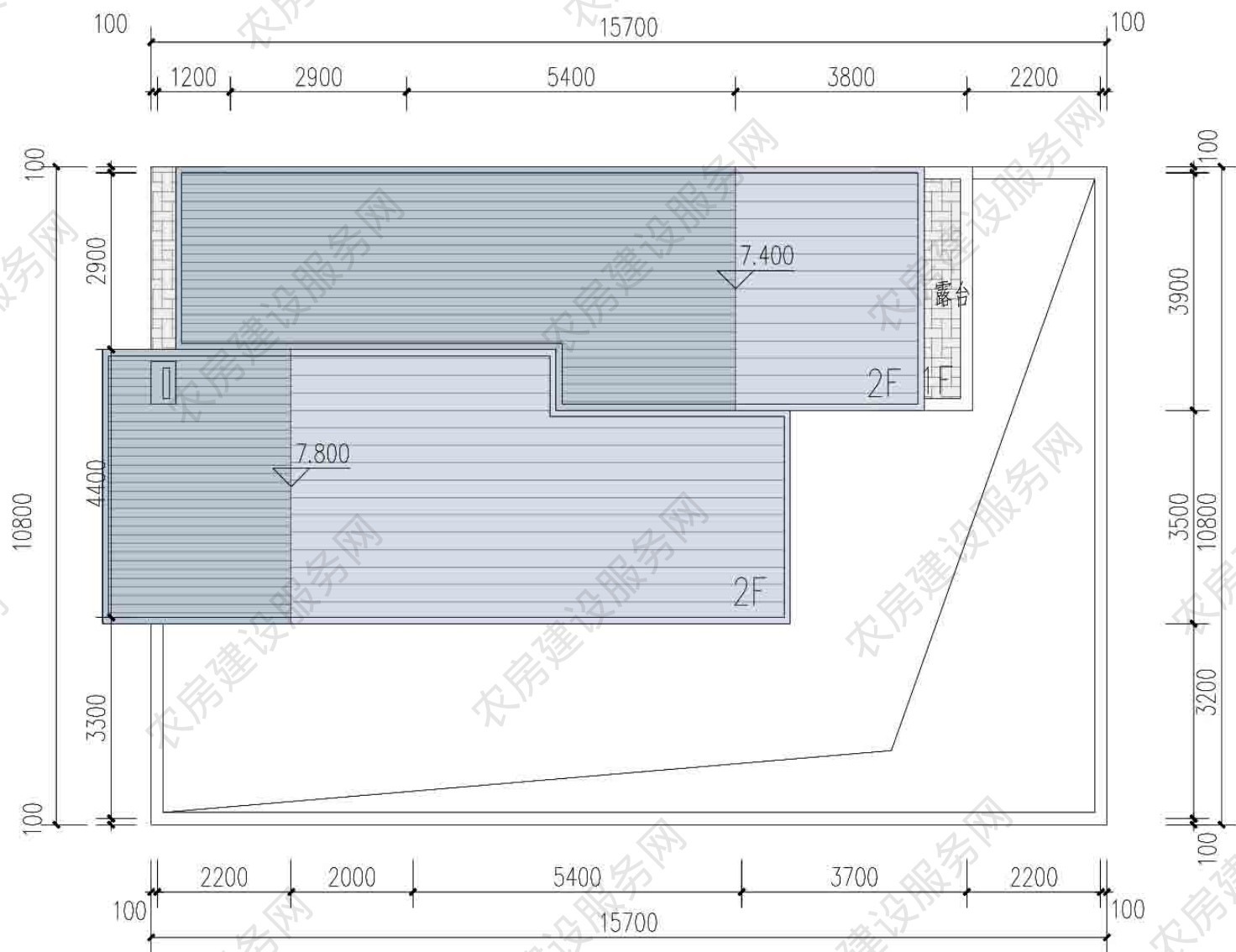
屋顶平面图
