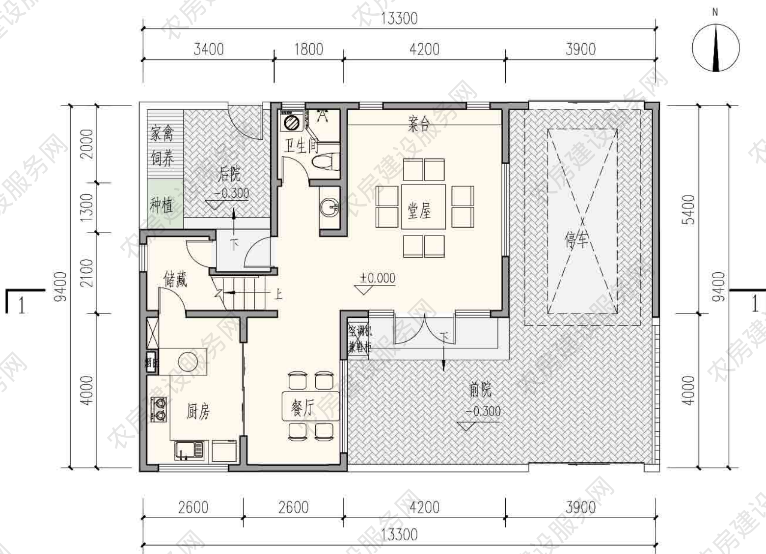
一层平面图
