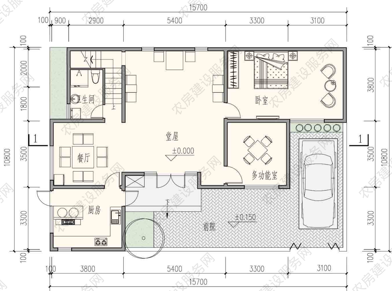
一层平面图
