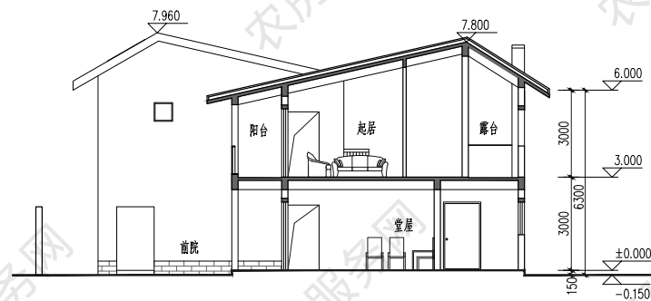
1-1 剖面图
