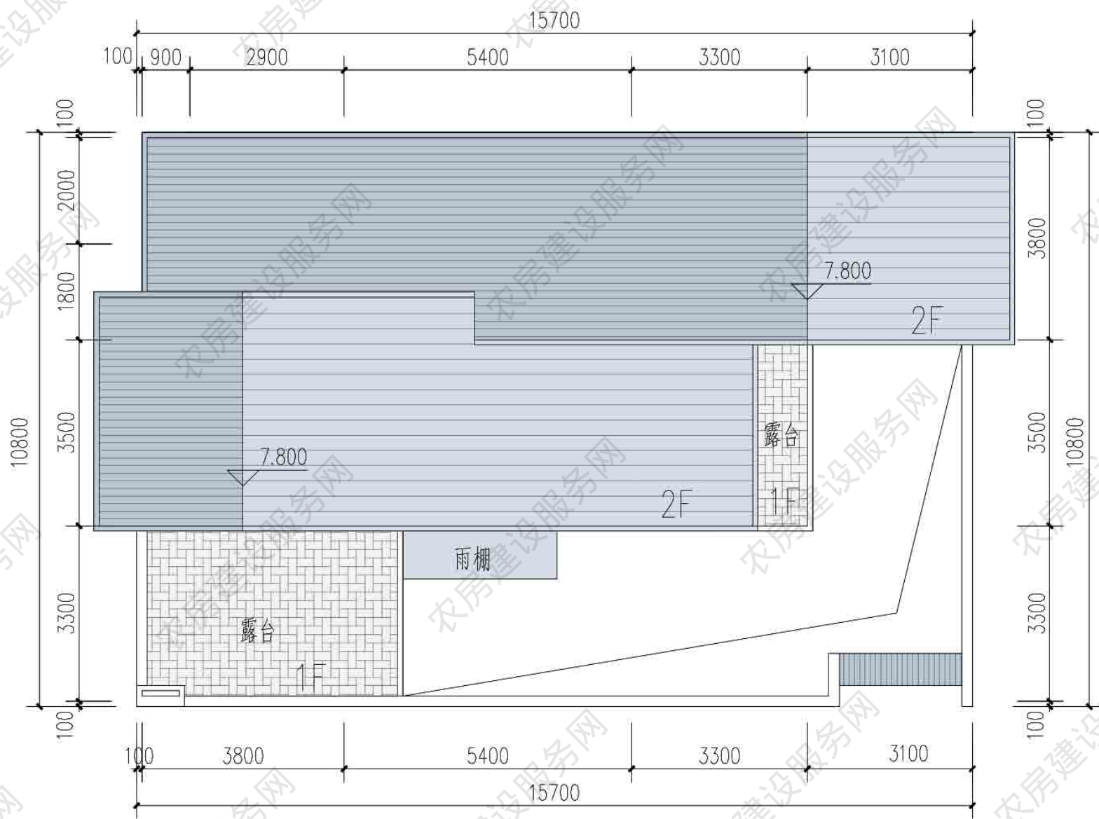
屋顶平面图
