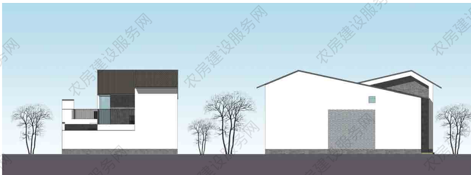
东立面图
