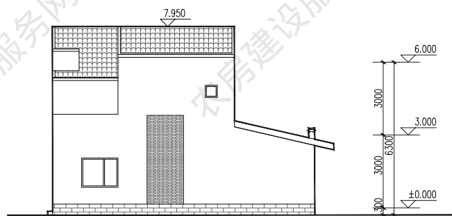
西立面图
