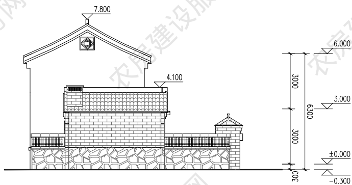
西立面图
