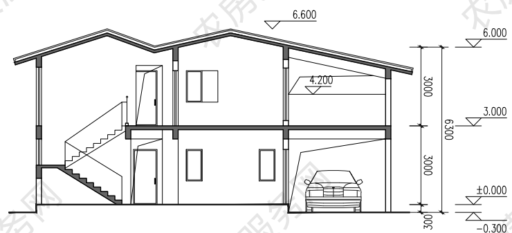
1-1 剖面图
