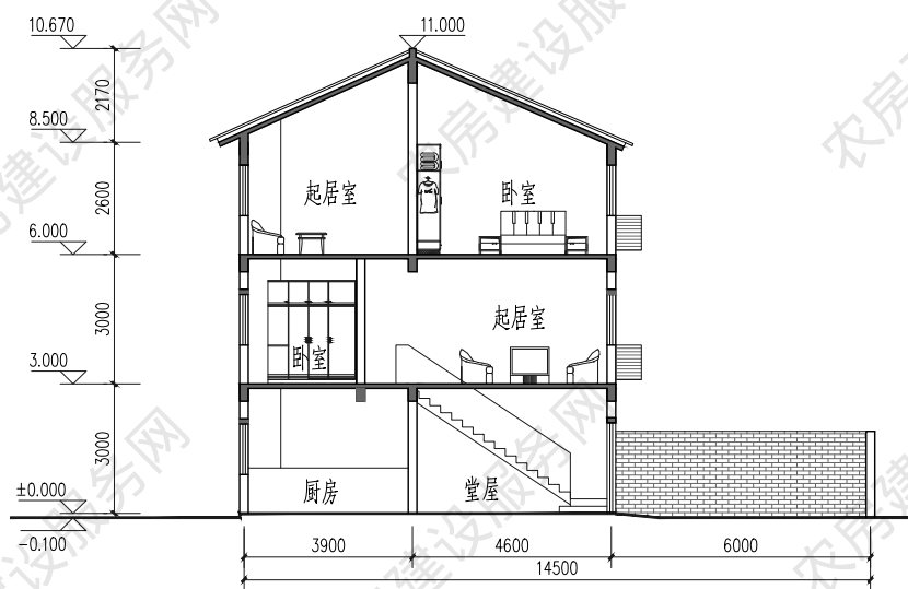
1-1 剖面图
