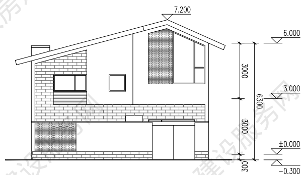
南立面图
