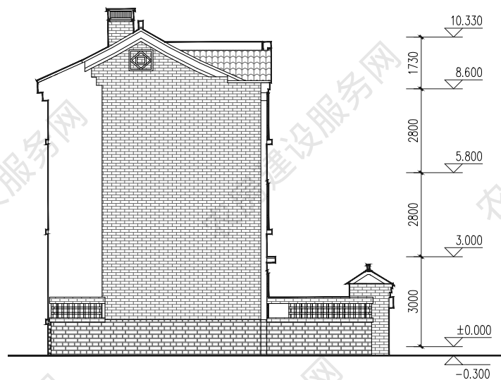
西立面图
