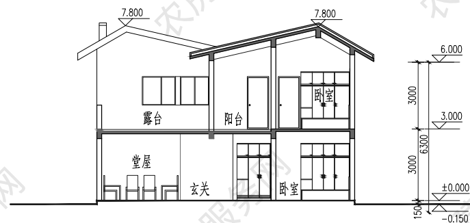
1-1 剖面图
