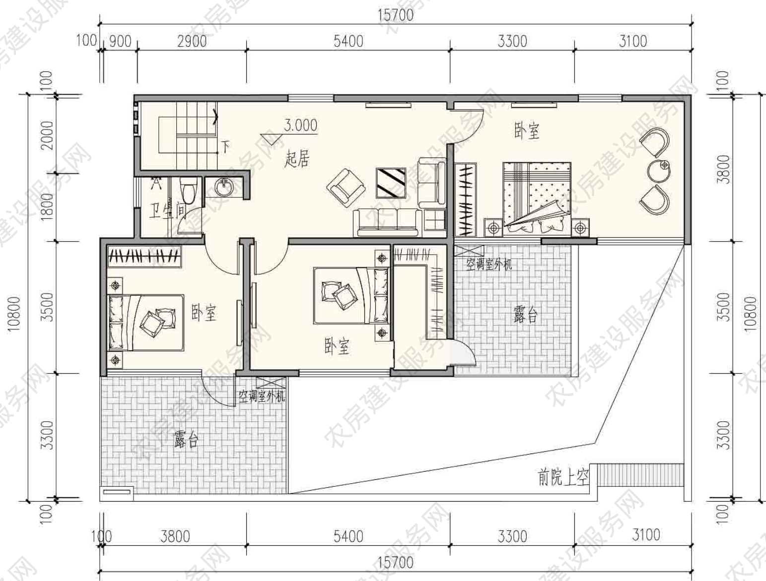
二层平面图
