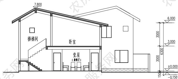
1-1 剖面图
