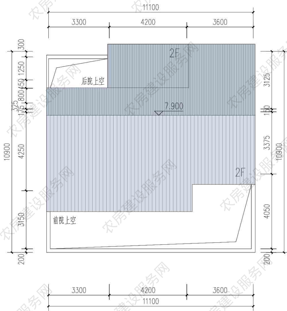
屋顶平面图
