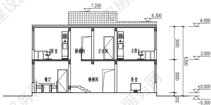
1-1 剖面图
