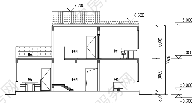
1-1 剖面图
