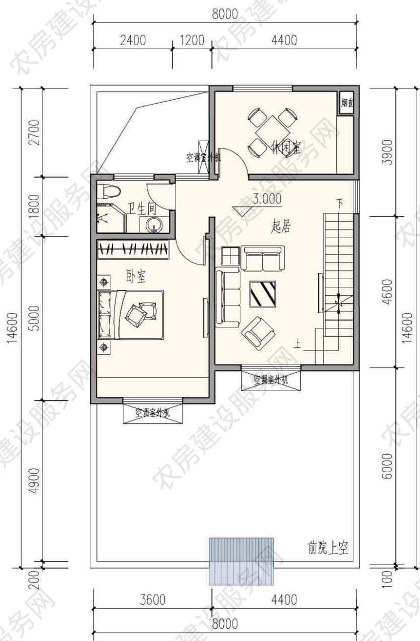
二层平面图
