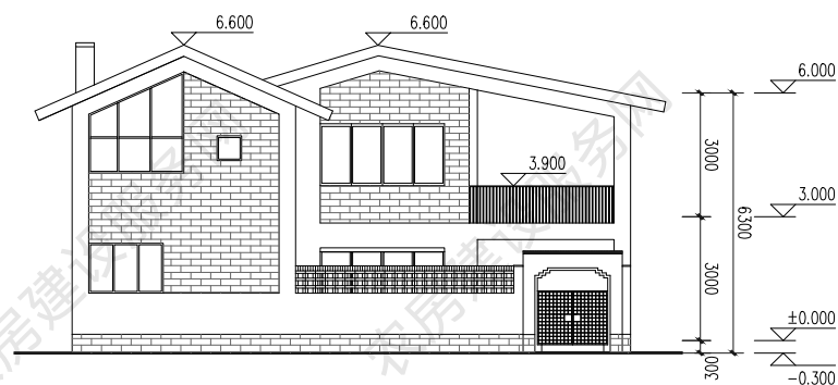
南立面图
