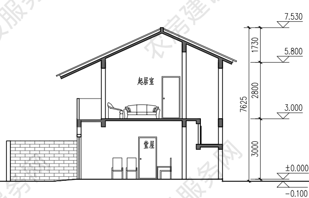
1-1 剖面图
