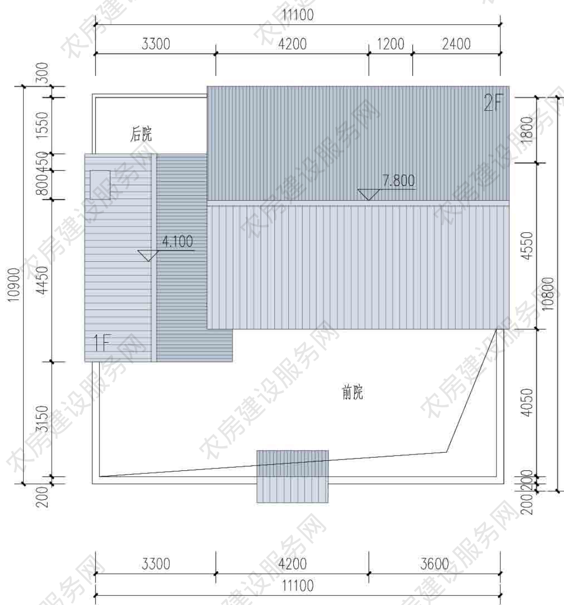
屋顶平面图
