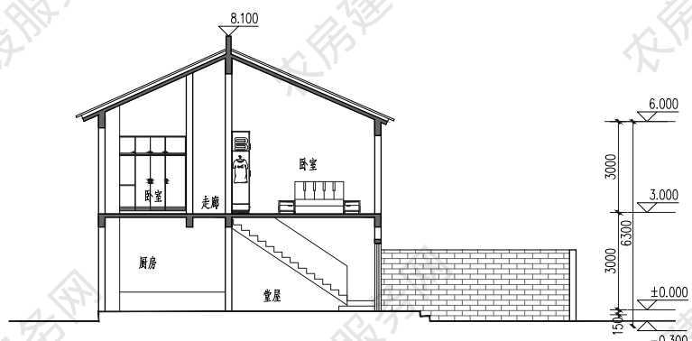
1-1 剖面图
