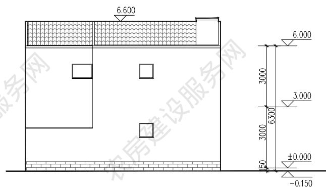
东立面图
