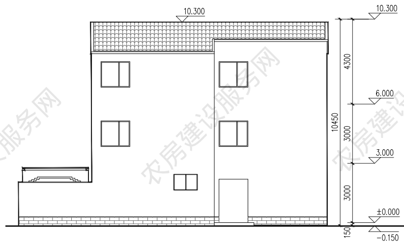
北立面图
