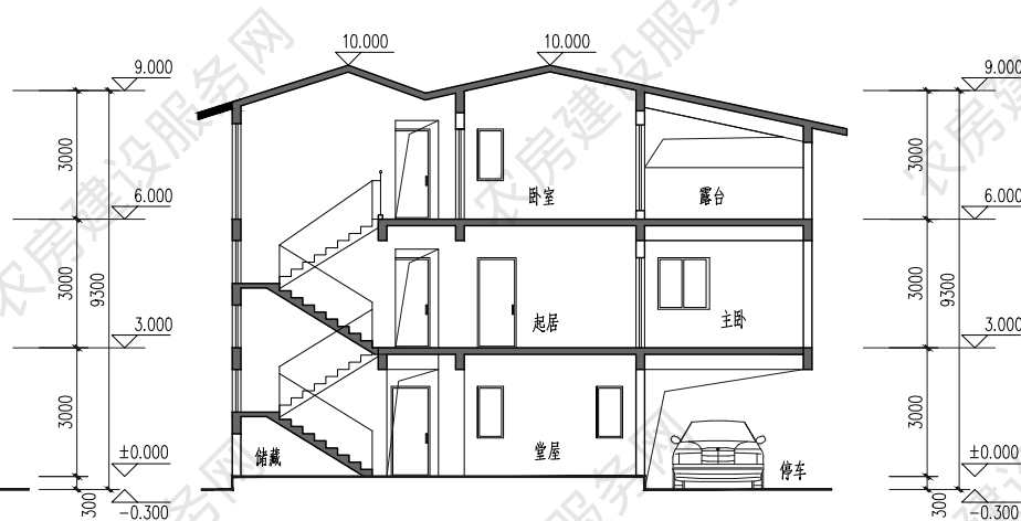
1-1 剖面图
