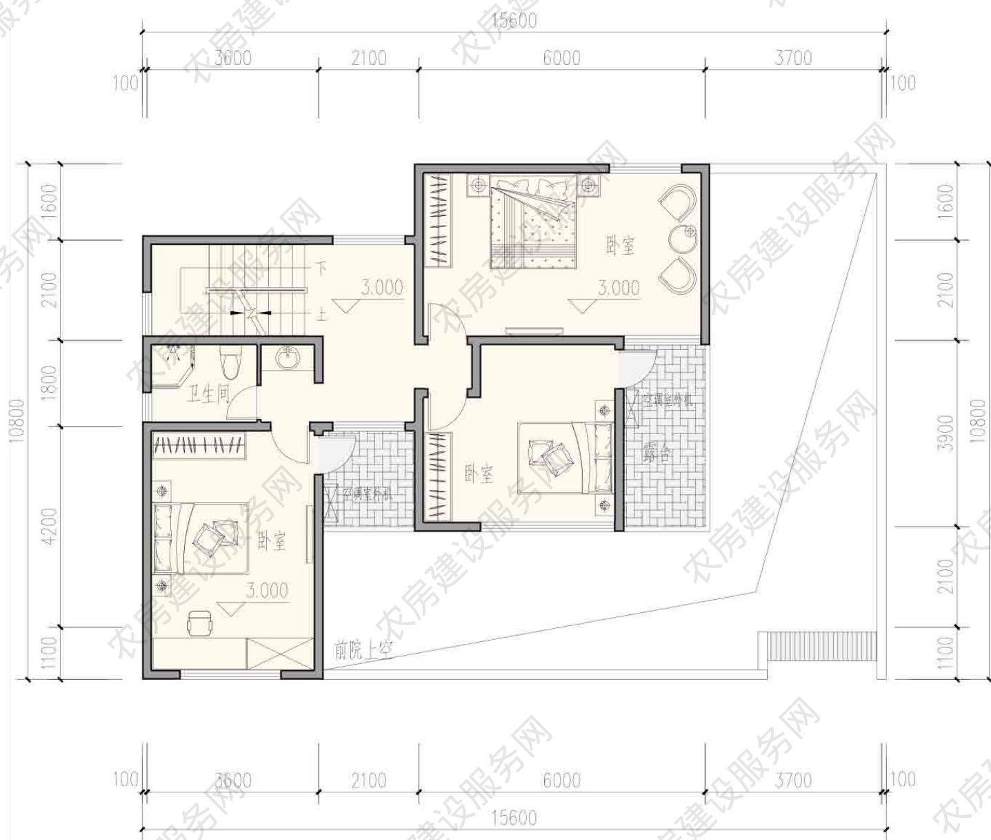
二层平面图 本层建筑面积 84 平方米
