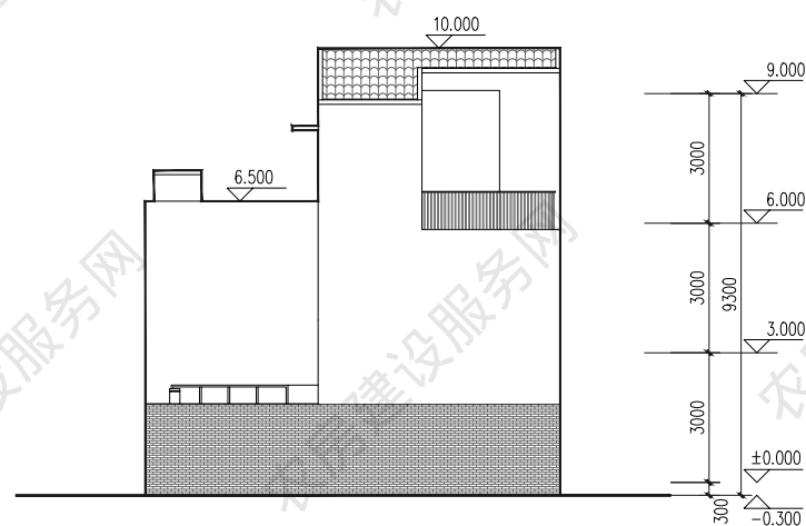
东立面图
