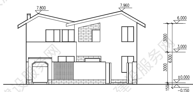
南立面图
