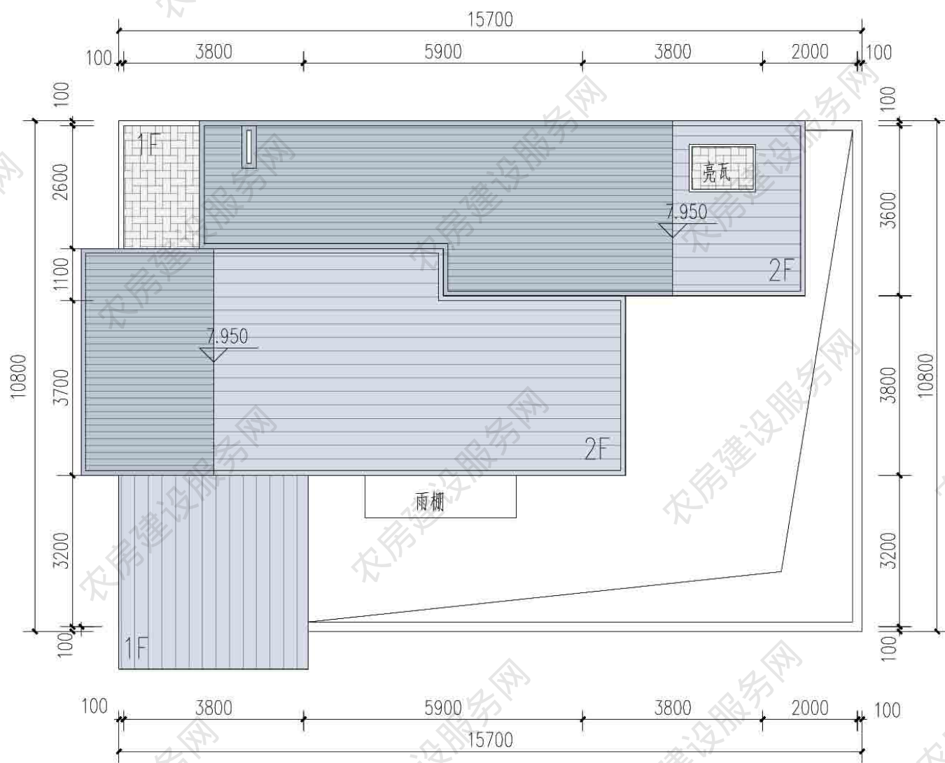
屋顶平面图
