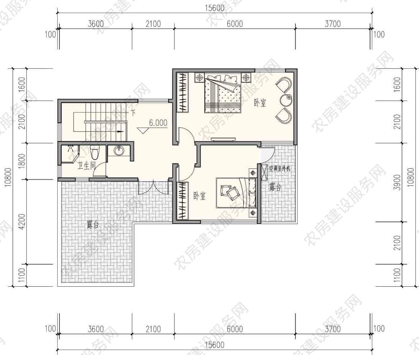
三层平面图
