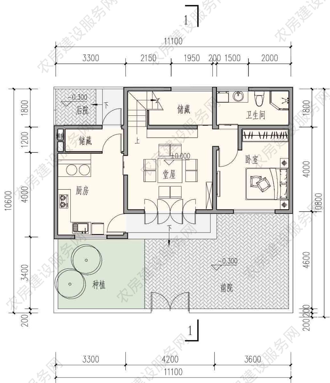
一层平面图 本层建筑面积 66 平方米
