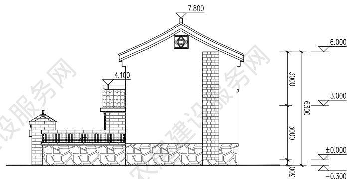
东立面图
