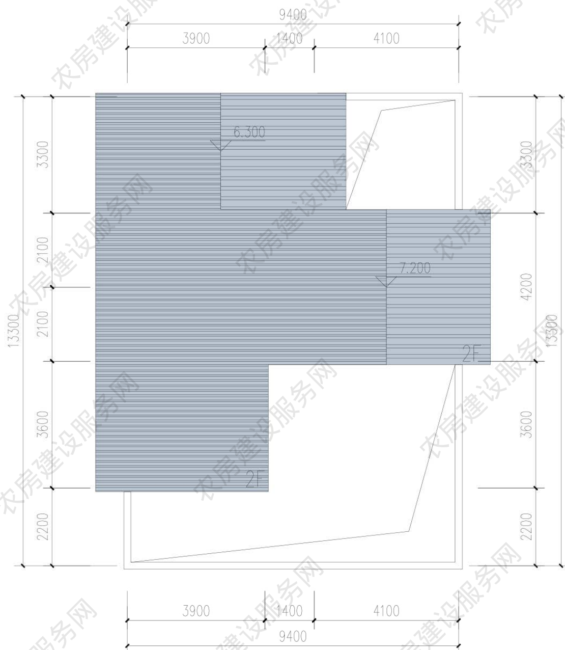
屋顶平面图
