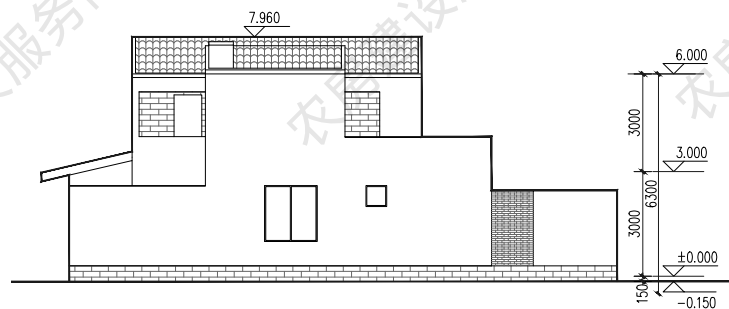
西立面图
