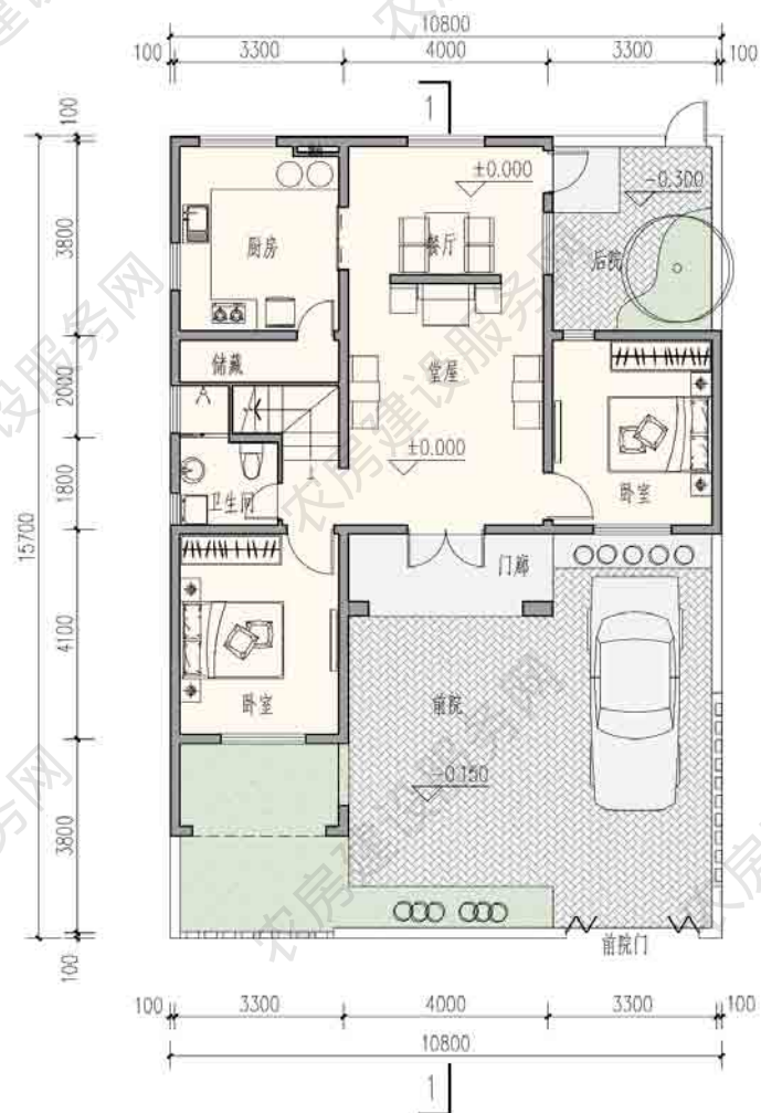
一层平面图 本层建筑面积 91 平方米
