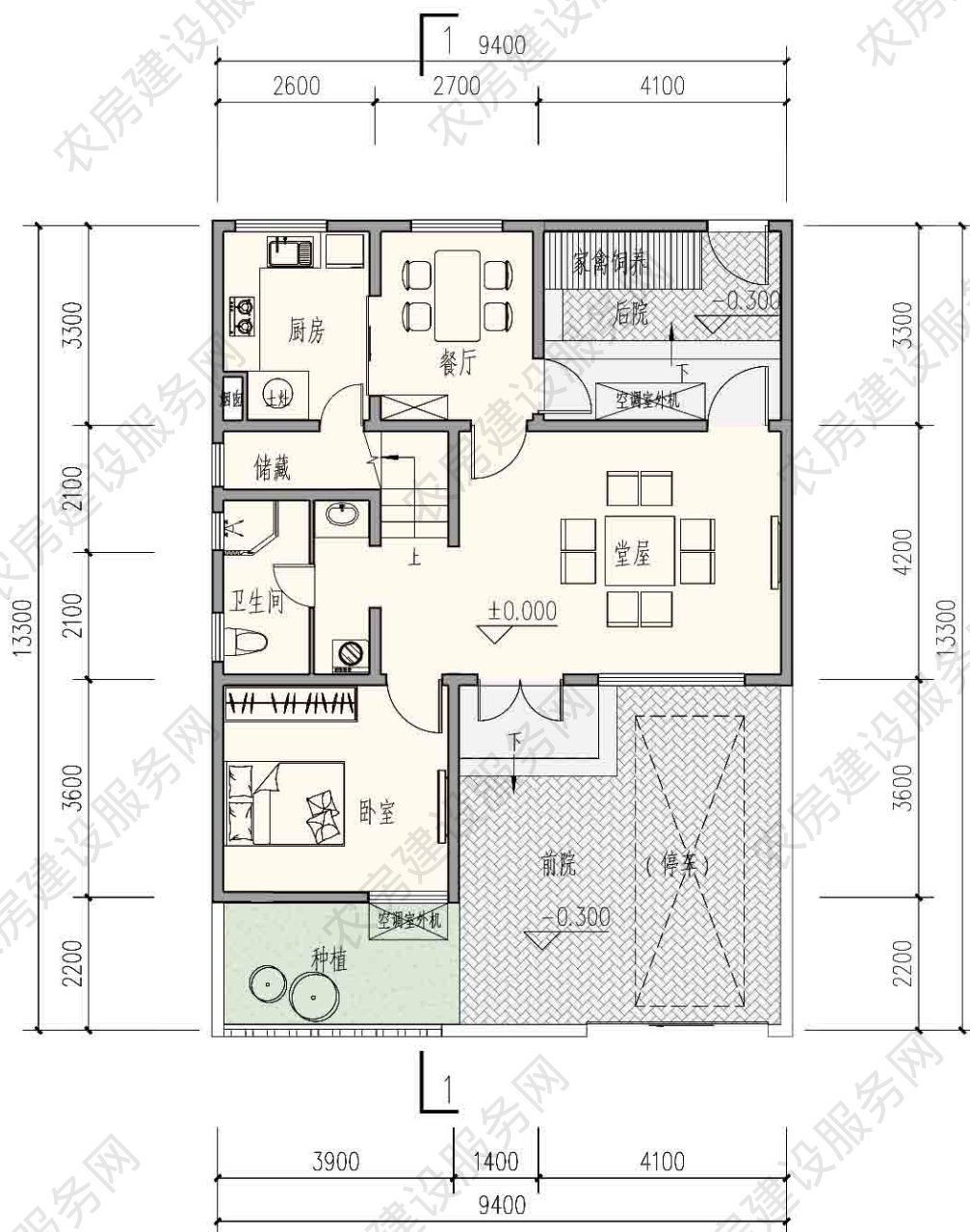
一层平面图 本层建筑面积 75 平方米
