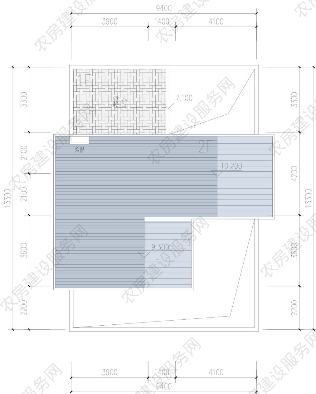
屋顶平面图
