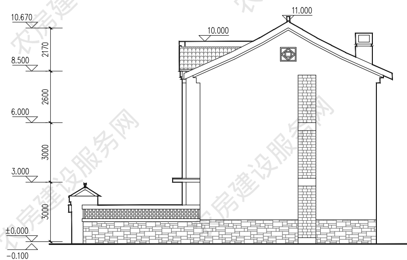
东立面图
