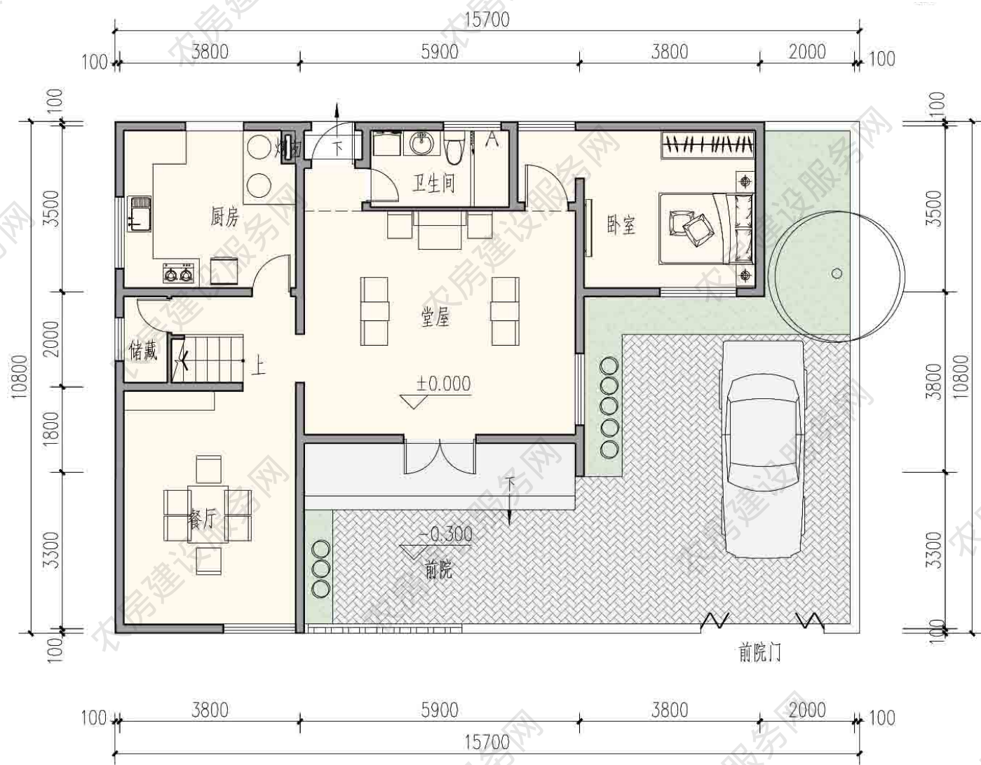
一层平面图
