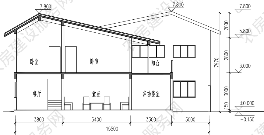
1-1 剖面图
