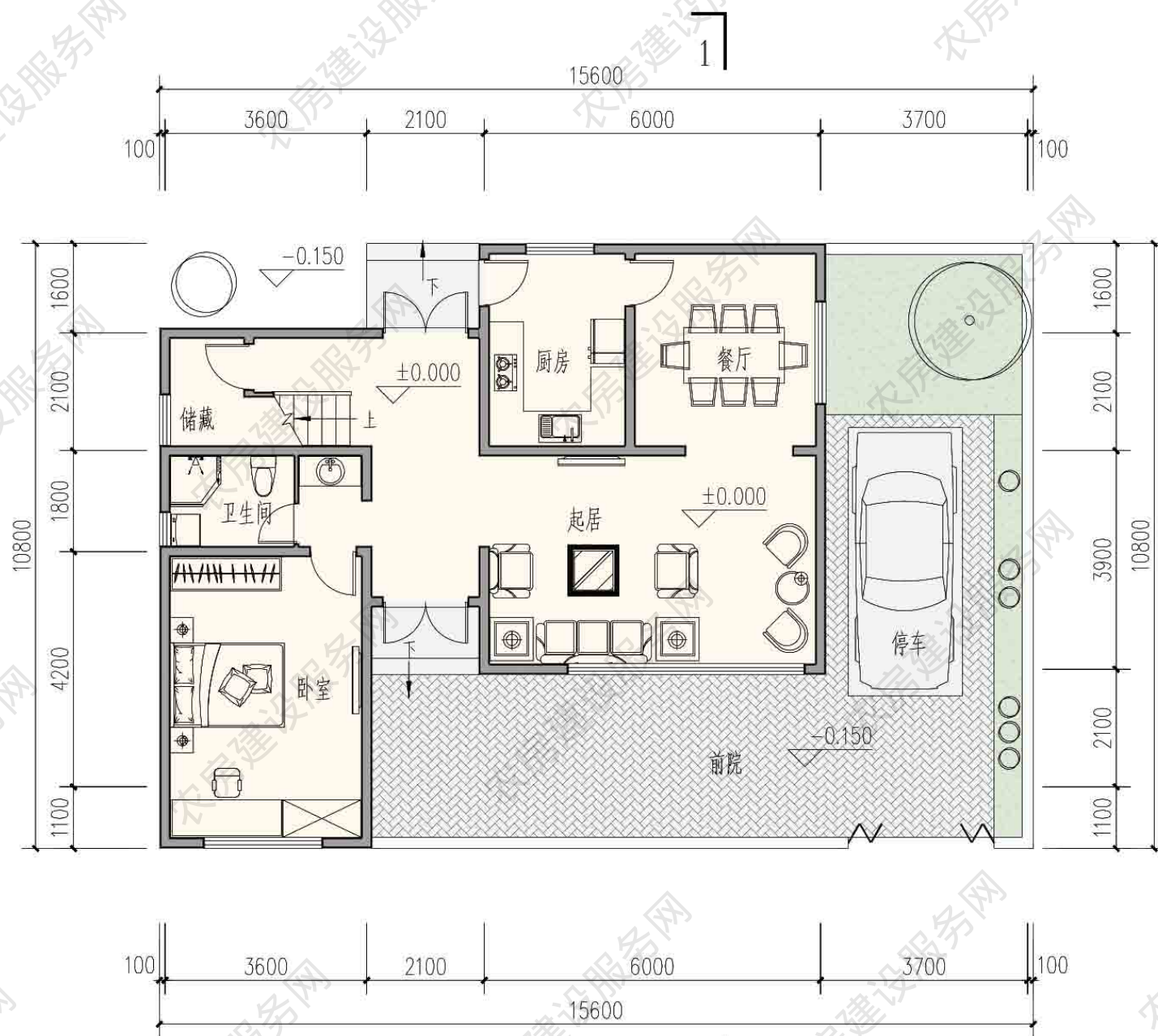
一层平面图
