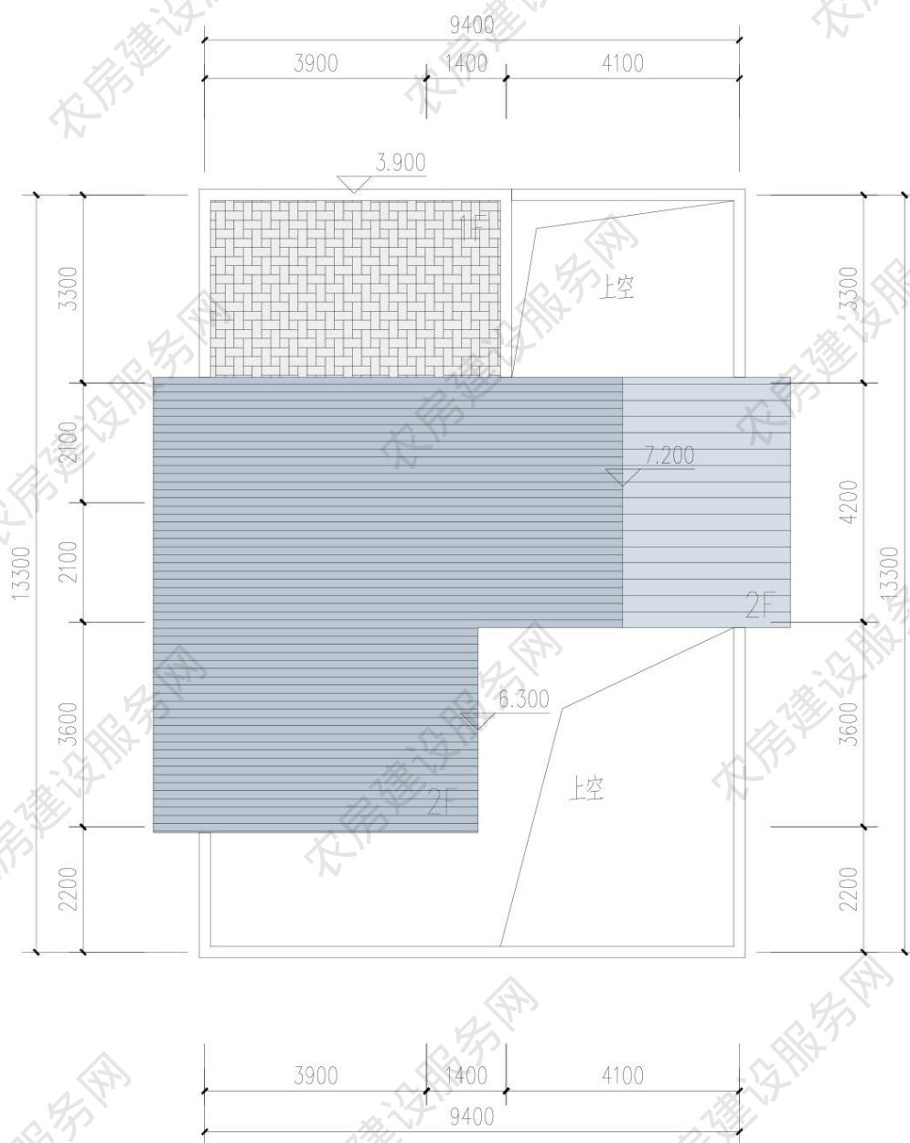
屋顶平面图
