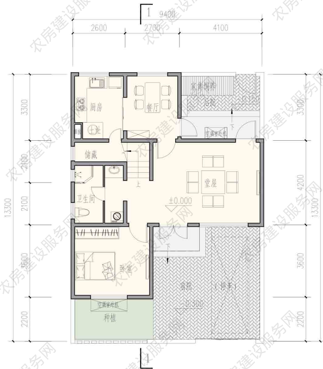
一层平面图 本层建筑面积 75 平方米
