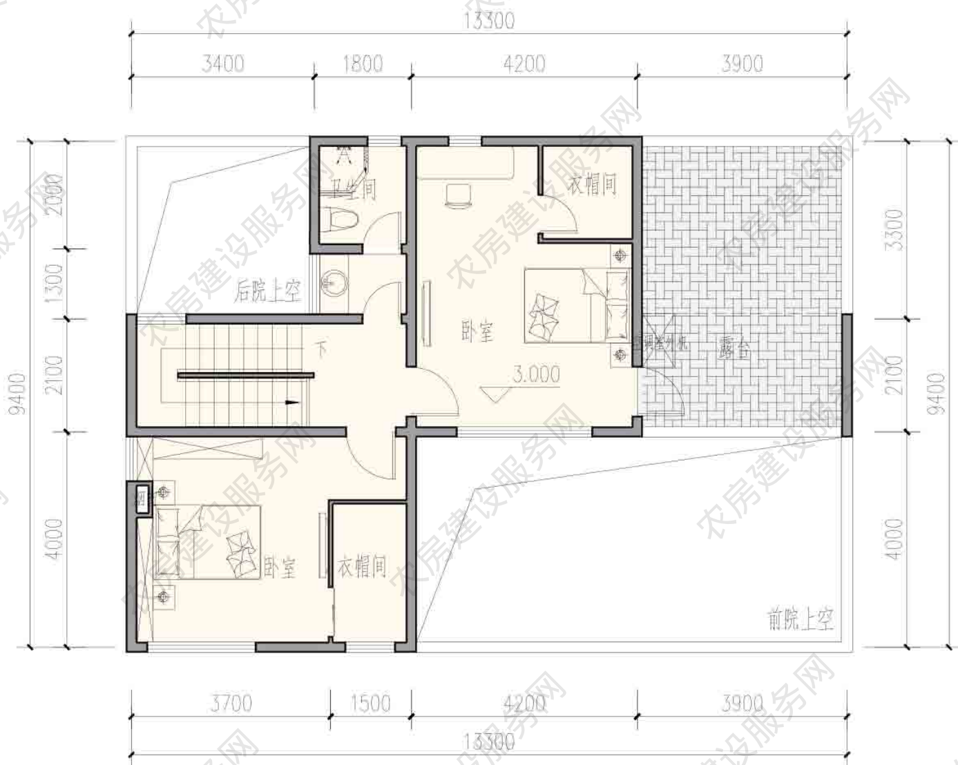
二层平面图
