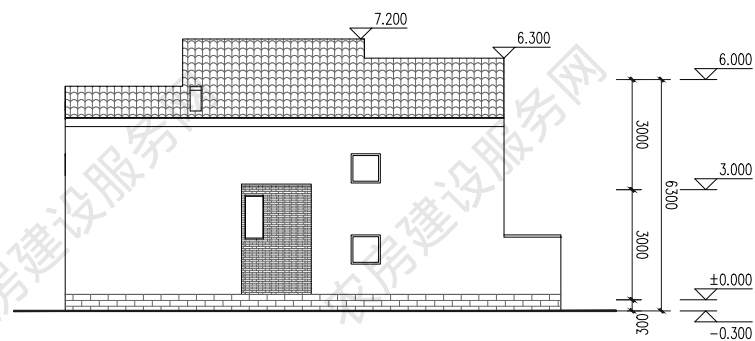
西立面图
