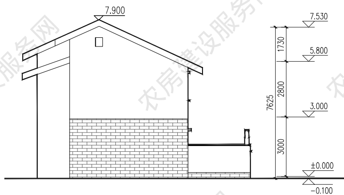
西立面图
